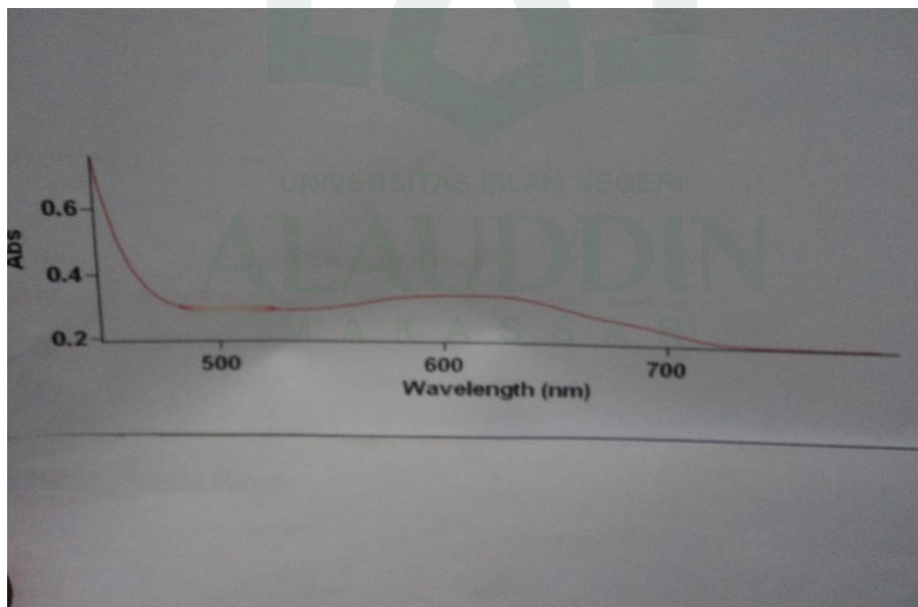
Gambar 6. Gambar hasil Spektrofotometer panjang gelombang Glukosa
