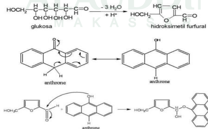
Gambar 5. Mekanisme Reaksi Anthrone dengan Glukosa
