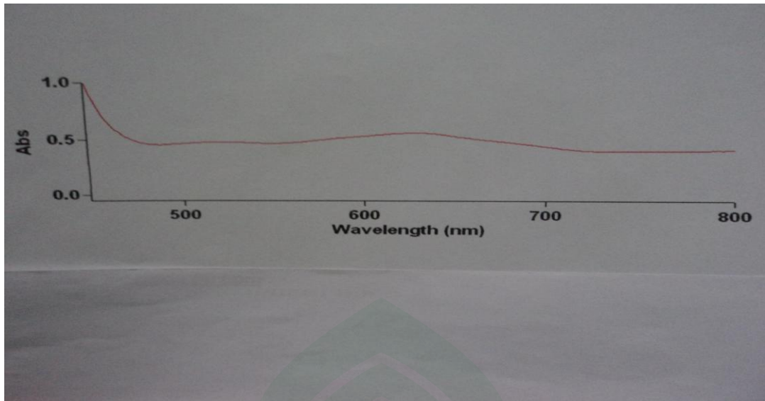
Gambar 7. Gambar hasil Spektrofotometer panjang gelombang Fruktosa
