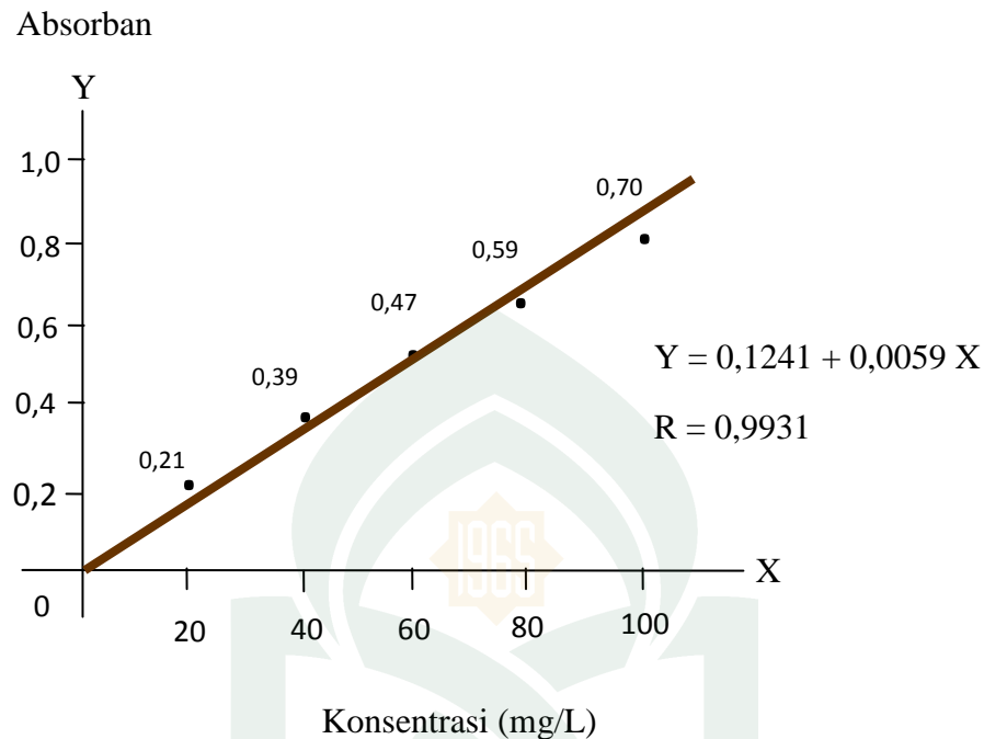
Gambar 4. Gambar perbandingan konsentasi glukosa dan absorbans pada panjang gelombang 628 nm.
