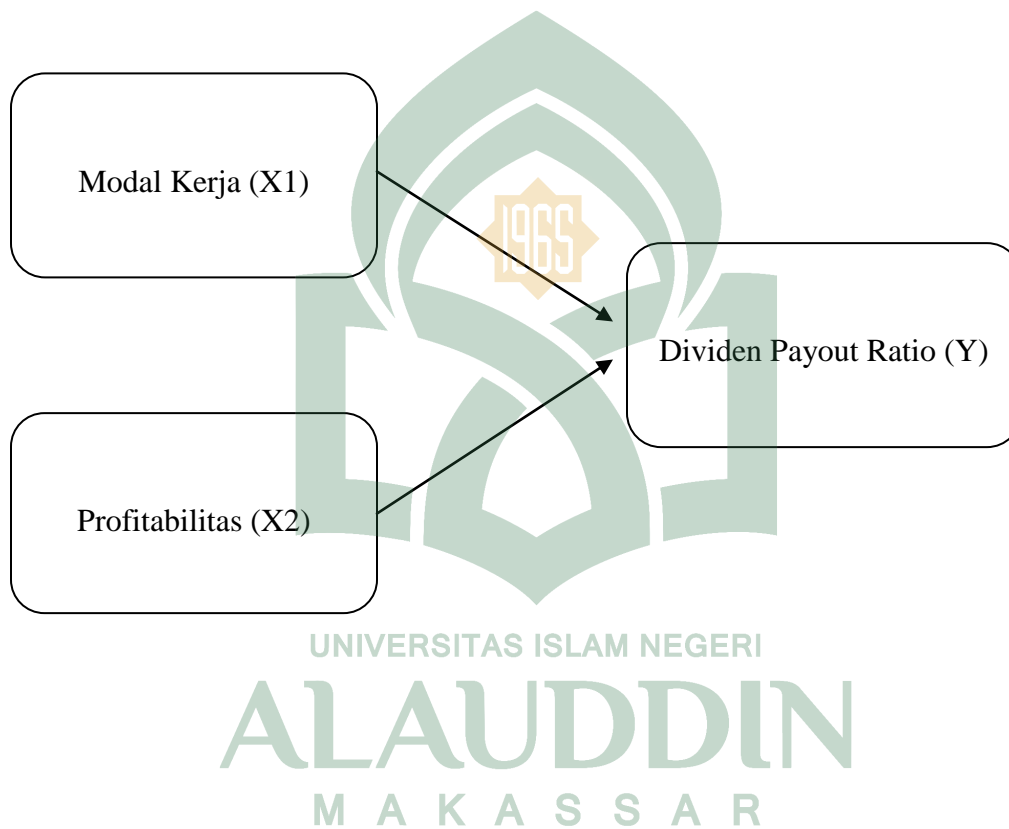
Gambar 2.1 Kerangka Konseptual
