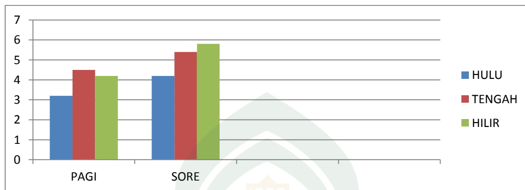
Grafik 5.3 Hasil Pengukuran Tingkat Pencemaran Air ditinjau dari Parameter BOD ( Biological Oxygen Demand ) di Badan Air Sungai Jeneberang di Kelurahan Pangkabinanga, Juni Tahun 2011.
