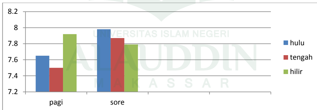
Grafik 5.2 Hasil Pengukuran Tingkat Pencemaran Air ditinjau dari Parameter pH (Power Hydrogen) di Badan Air Sungai Jeneberang di Kelurahan Pangkabinanga, Juni Tahun 2011.
