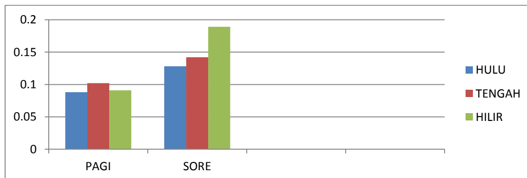
Grafik 5.1 Hasil Pengukuran Tingkat Pencemaran Air ditinjau dari Parameter Kadar Timbal ( Pb ) di Badan Air Sungai Jeneberang di Kelurahan Pangkabinanga, Juni Tahun 2011.
