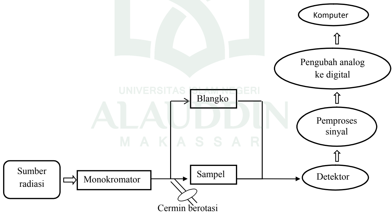
Gambar 3. Skema kerja spektrofotometer UV-Vis (Mulja, 1995).
