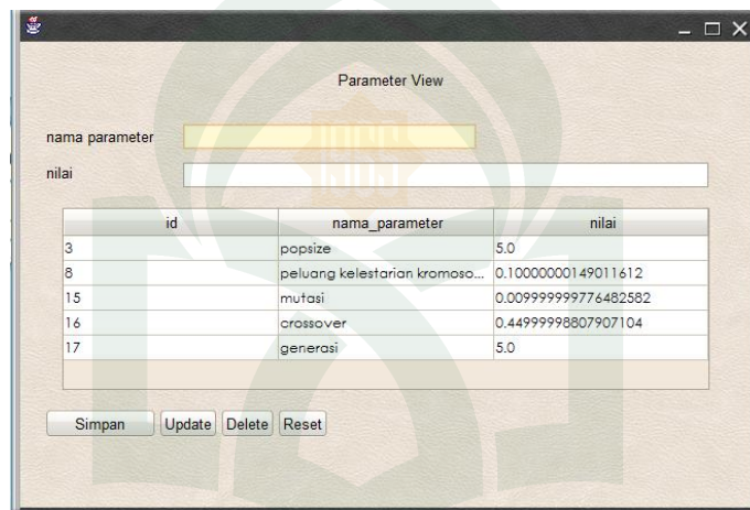
Gambar V. 6. Interface Parameter
