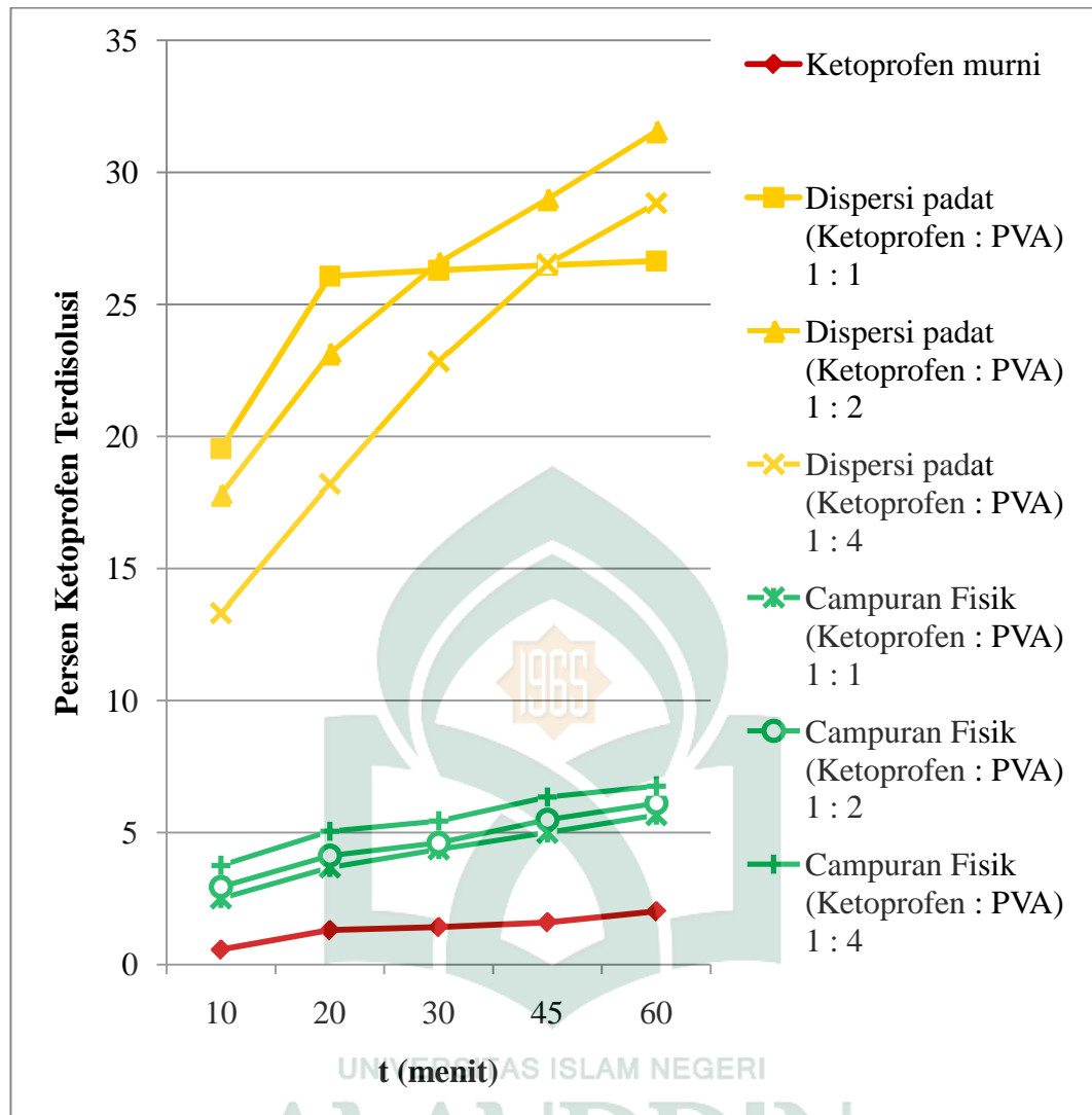
Gambar 8. Hubungan kadar ketoprofen terdisolusi (%) dengan waktu (menit)
