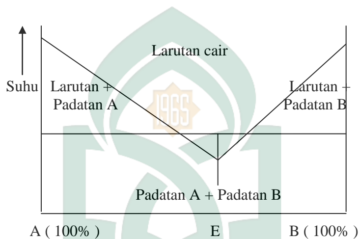
Gambar 1. Diagram fase campuran eutektikum sederhana dengan kelarutan padat yang diabaikan (Chiou, 1971)
