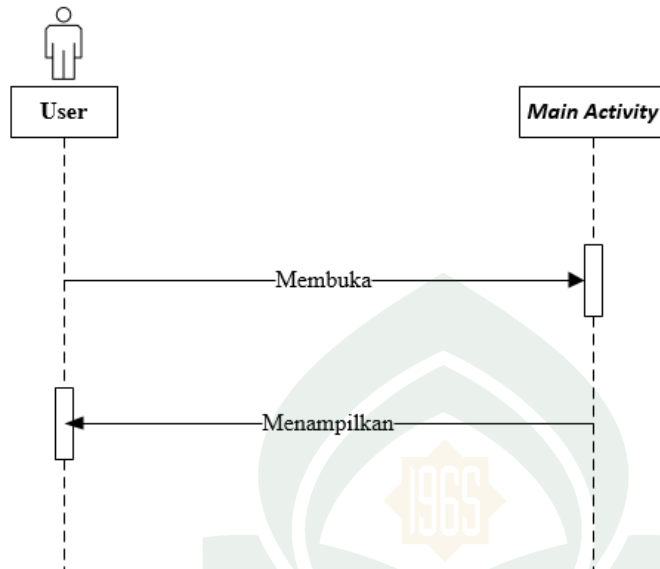
Gambar IV. 5. Sequence Diagram untuk Membuka Aplikasi
