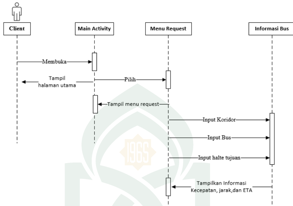
Gambar IV. 7. Sequence Diagram untuk Melakukan request data
