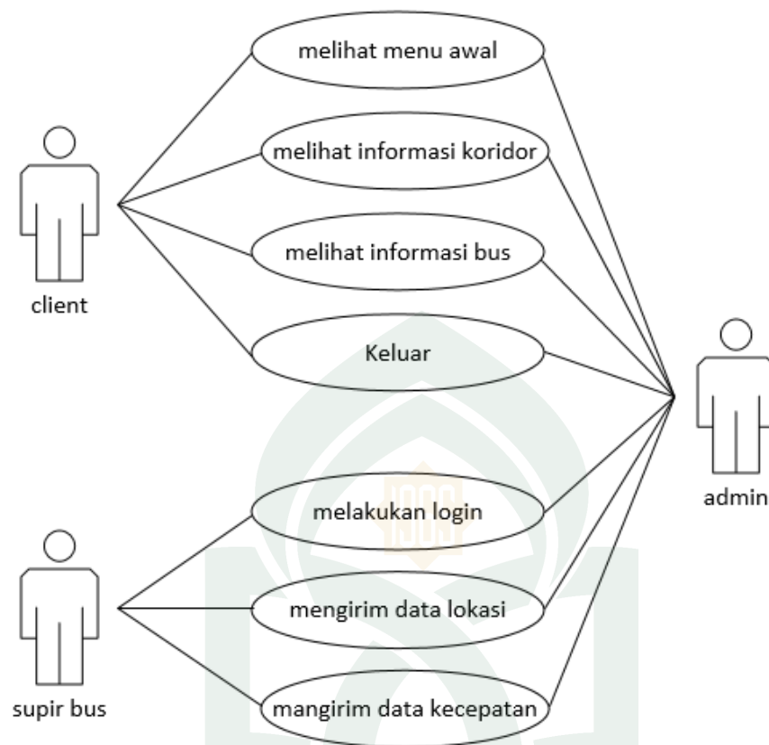
Gambar IV. 3. Use Case Diagram Sistem yang Diusulkan
