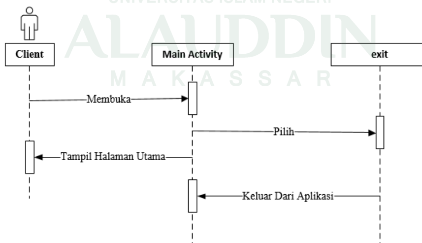
Gambar IV.8 Sequence Diagram keluar dari Aplikasi.
