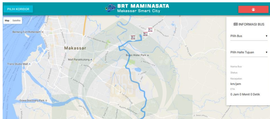
Gambar V.2 Hasil perancangan form utama
