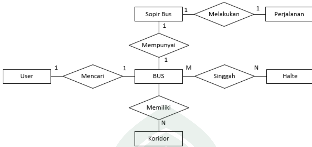
Gambar IV. 2. ERD pada server.
