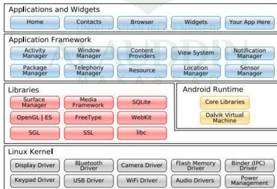
Gambar II. 7 Arsitektur Android, Safaat (2014).
