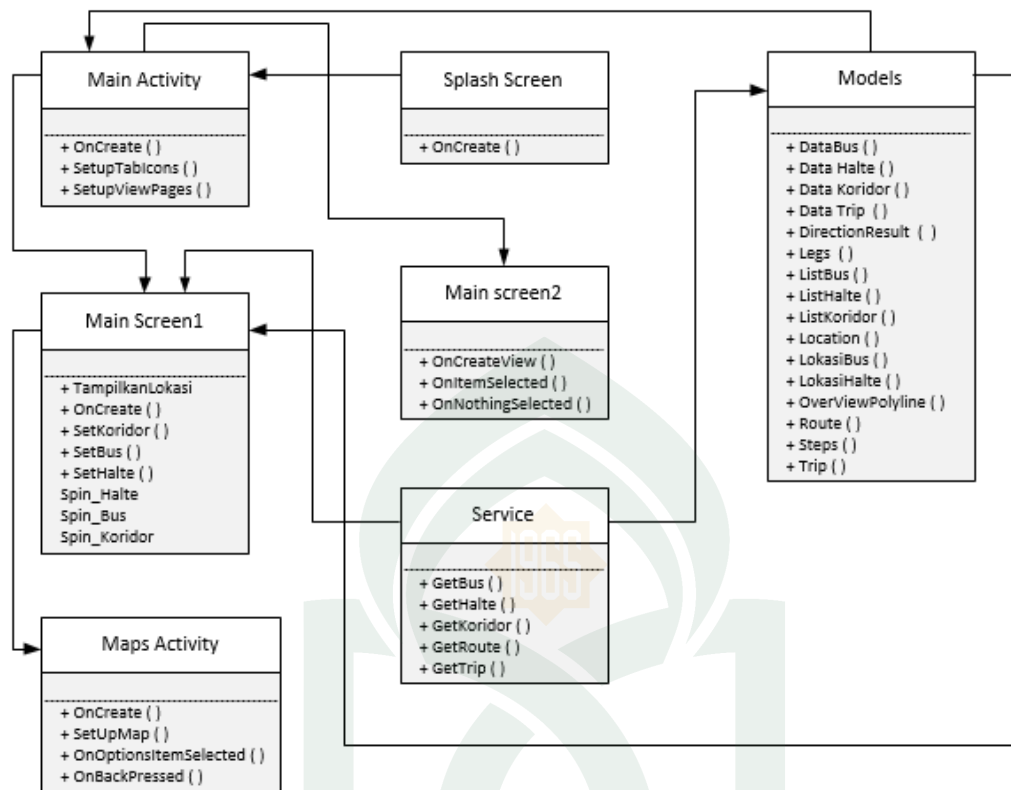
Gambar IV. 4. Class Diagram Sistem yang Diusulkan
