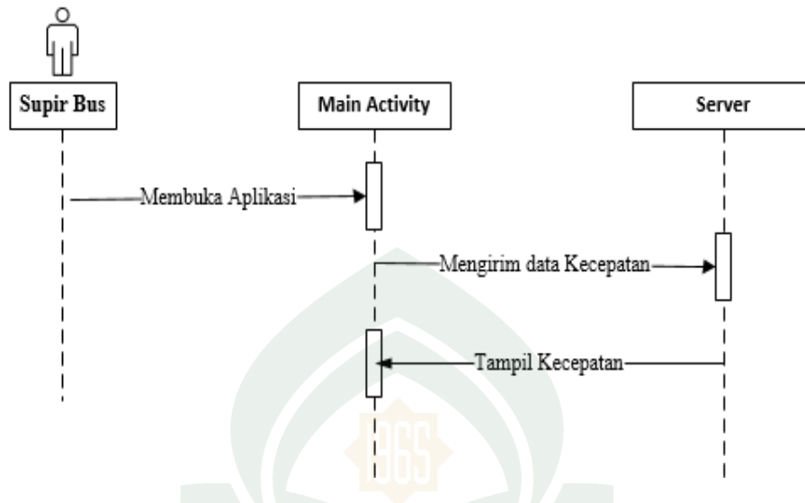
Gambar IV. 11. Sequence Diagram untuk Mengirim data kecepatan bus ke server
