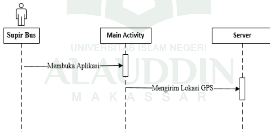
Gambar IV. 10. Sequence Diagram untuk mengirim data lokasi bus ke server
