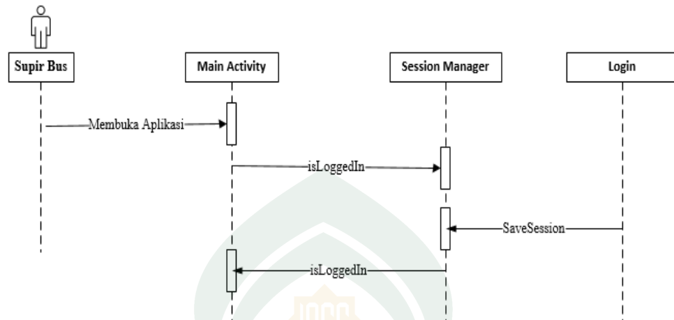
Gambar IV. 9. Sequence Diagram untuk melakukan login supir Bus
