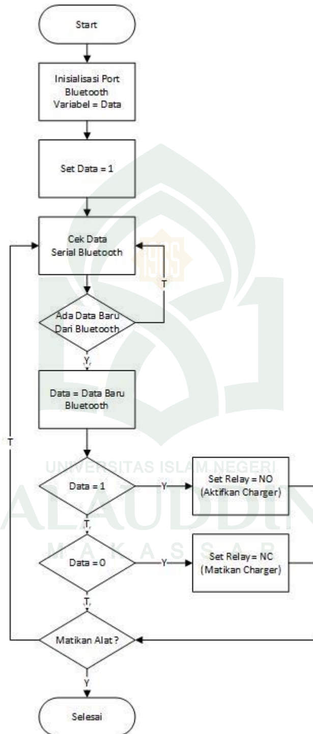
Gambar IV.4 Flowchart Alat Pada Arduino.
