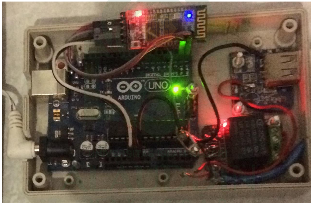
Gambar V.1 Hasil Rancangan Alat Smart Charger
