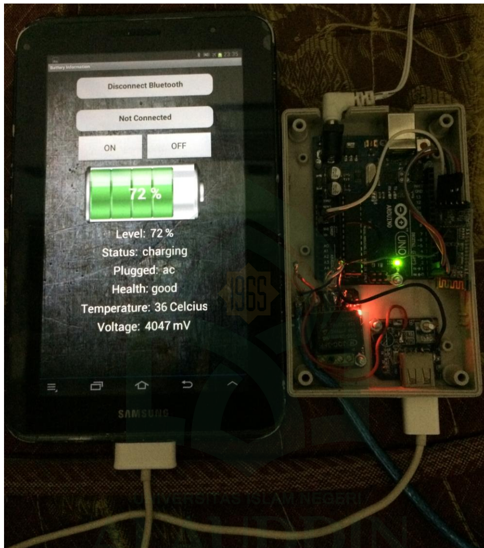
Gambar V.9 Alat smart charger dalam kondisi menyala
