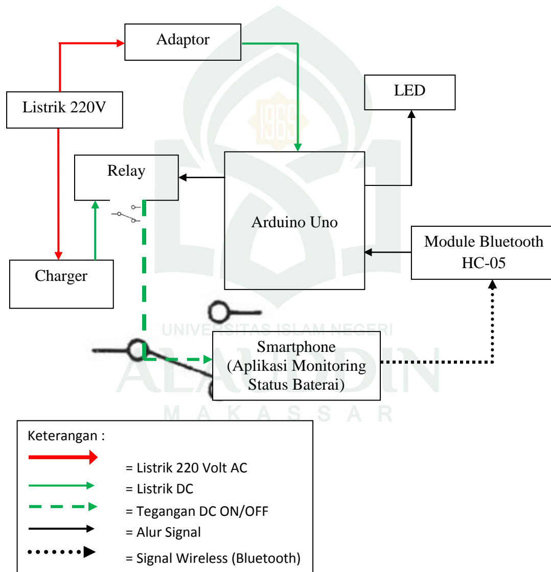
Gambar IV.1 Diagram Blok Perancangan Alat Smart Charger Pada Smartphone Menggunakan Arduino terdiri dari beberapa masukan dan keluaran.
