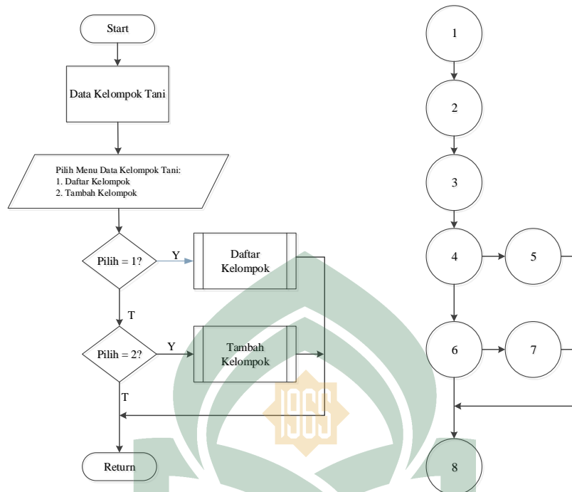
Gambar V.23 Flowchart dan Flowgraph Menu Anggota Kelompok Tani.
