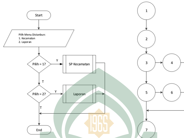
Gambar V.25 Flowchart dan Flowgraph Menu Utama Distanbun
