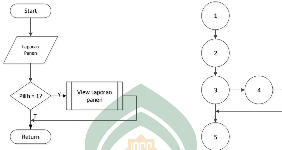
Gambar V.27 Flowchart dan Flowgraph Menu Laporan Panen
