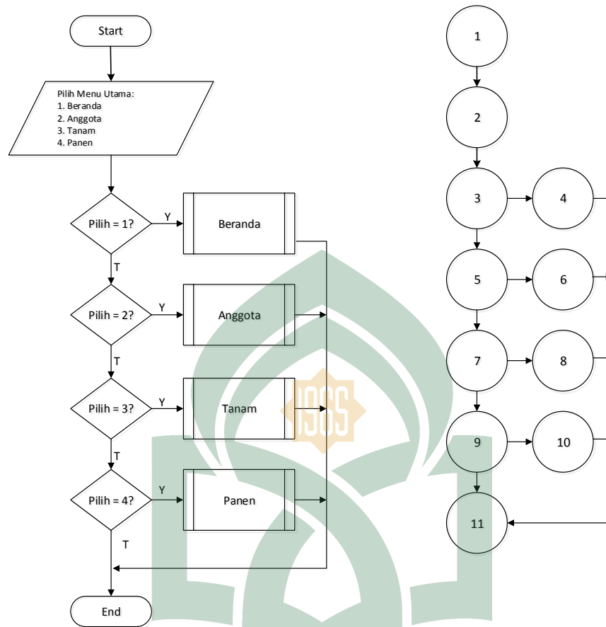
Gambar V.18 Flowchart dan Flowgraph Menu Utama pada Petani
