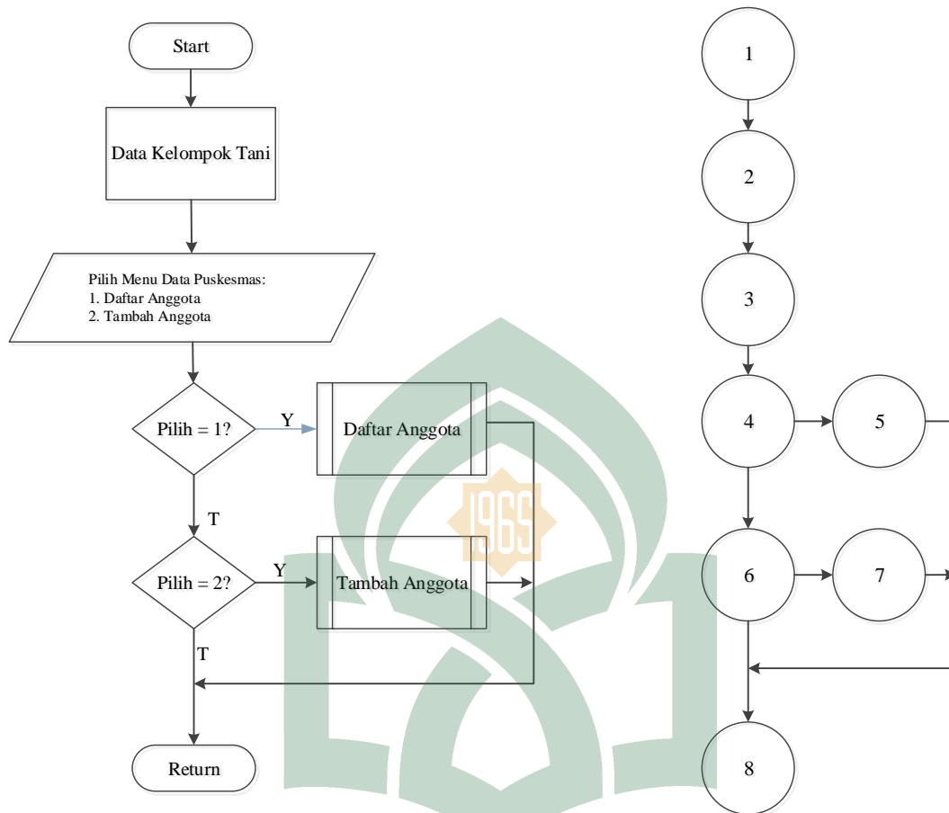
Gambar V.26 Flowchart dan Flowgraph Menu Anggota SP Kecamatan.
