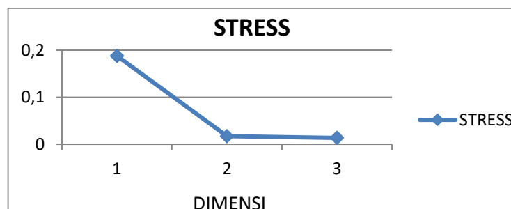
Gambar 4.4 Grafik nilai stress
