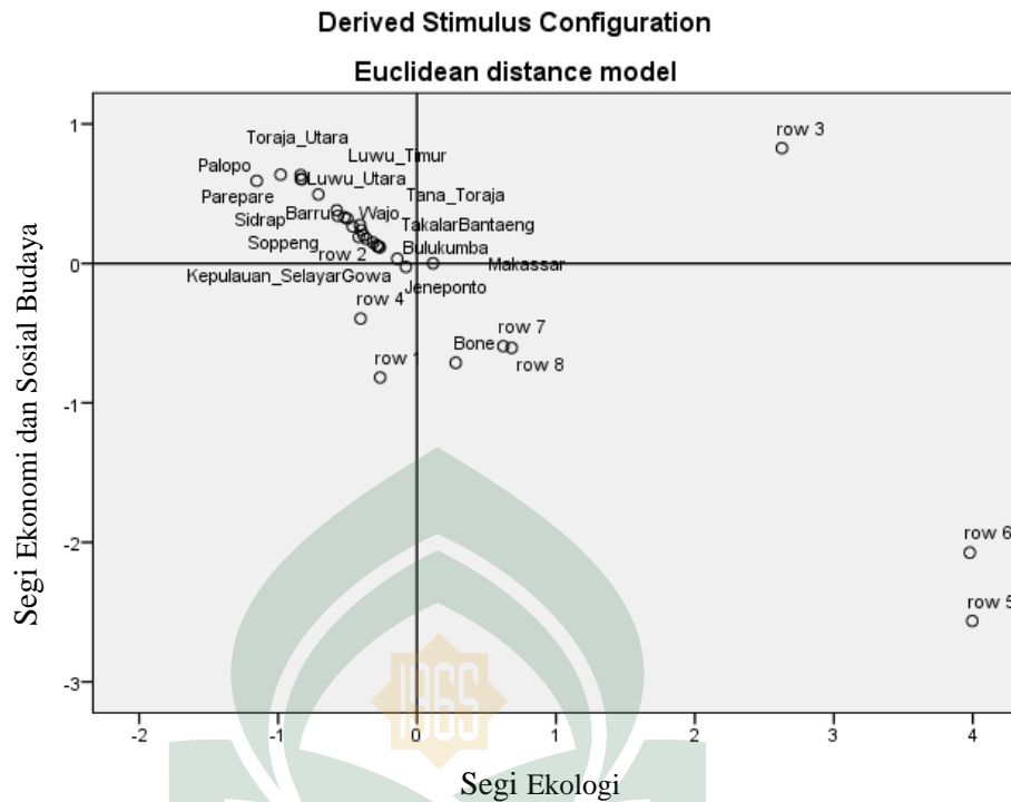
Gambar 4.7 Penamaan Dimensi pada Peta Spasial stimulus configuration Euclidean distance model
