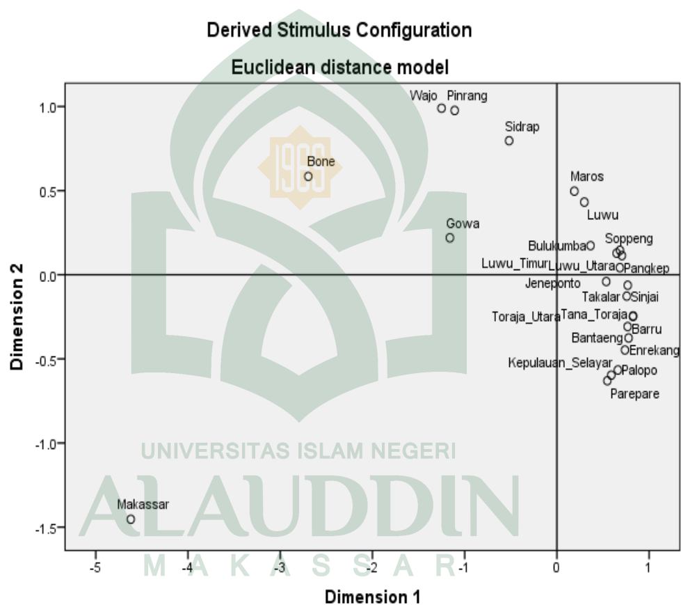
Gambar 4.5 Peta Spasial stimulus configuration Euclidean distance model untuk setiap objek
