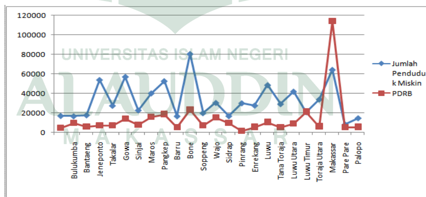
Gambar 4.2 Grafik Segi Ekonomi
