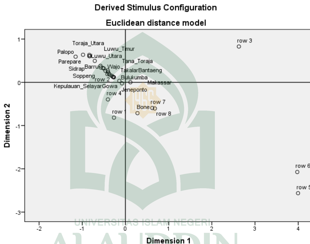
Gambar 4.6 Peta Spasial stimulus configuration Euclidean distance model untuk setiap objek dan variabelnya
