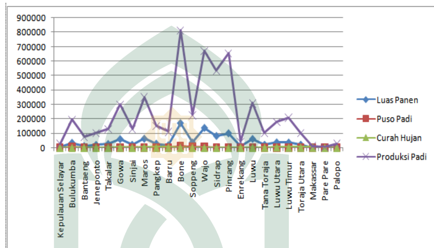
Gambar 4.1 Grafik Segi Ekologi
