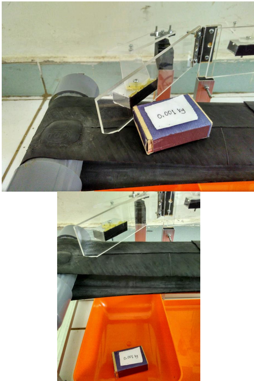
Gambar V. 8 Pensortiran pada Berat 0,001 Kg ( 1 gram).
