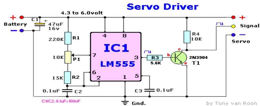
Gambar IV. 4 Rangkaian Motor Servo (Yudi, 2015 ).
