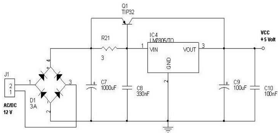
Gambar IV. 3 Rangkaian Power Supply (Suhartono, 2015).
