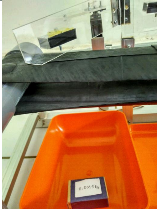
Gambar V. 13 Pensortiran pada Berat 0,0015 Kg ( 1,5 gram).
