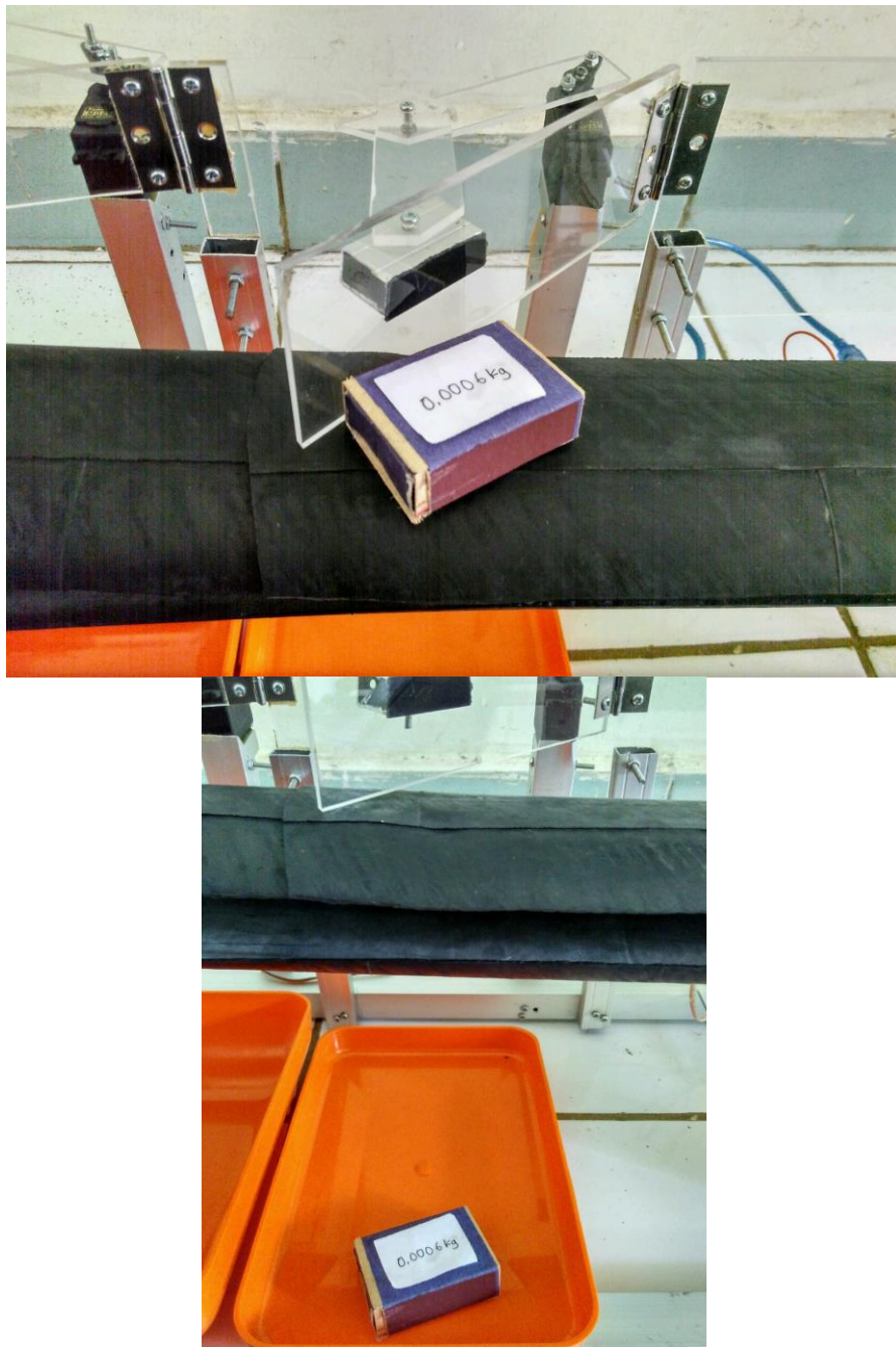
Gambar V. 4 Pensortiran pada Berat 0,0006 Kg (0,6 gram).
