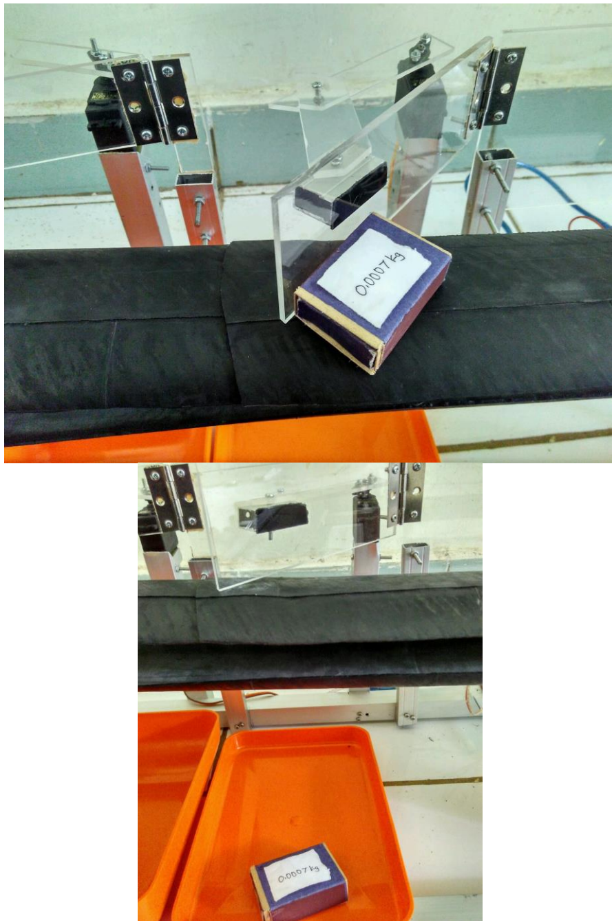
Gambar V. 5 Pensortiran pada Berat 0,0007 Kg (0,7 gram).
