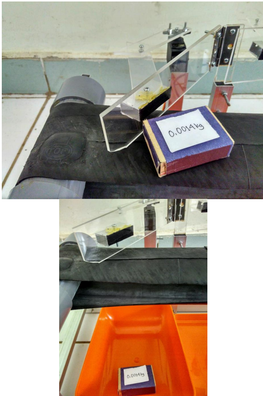
Gambar V. 12 Pensortiran pada Berat 0,0014 Kg ( 1,4 gram).
