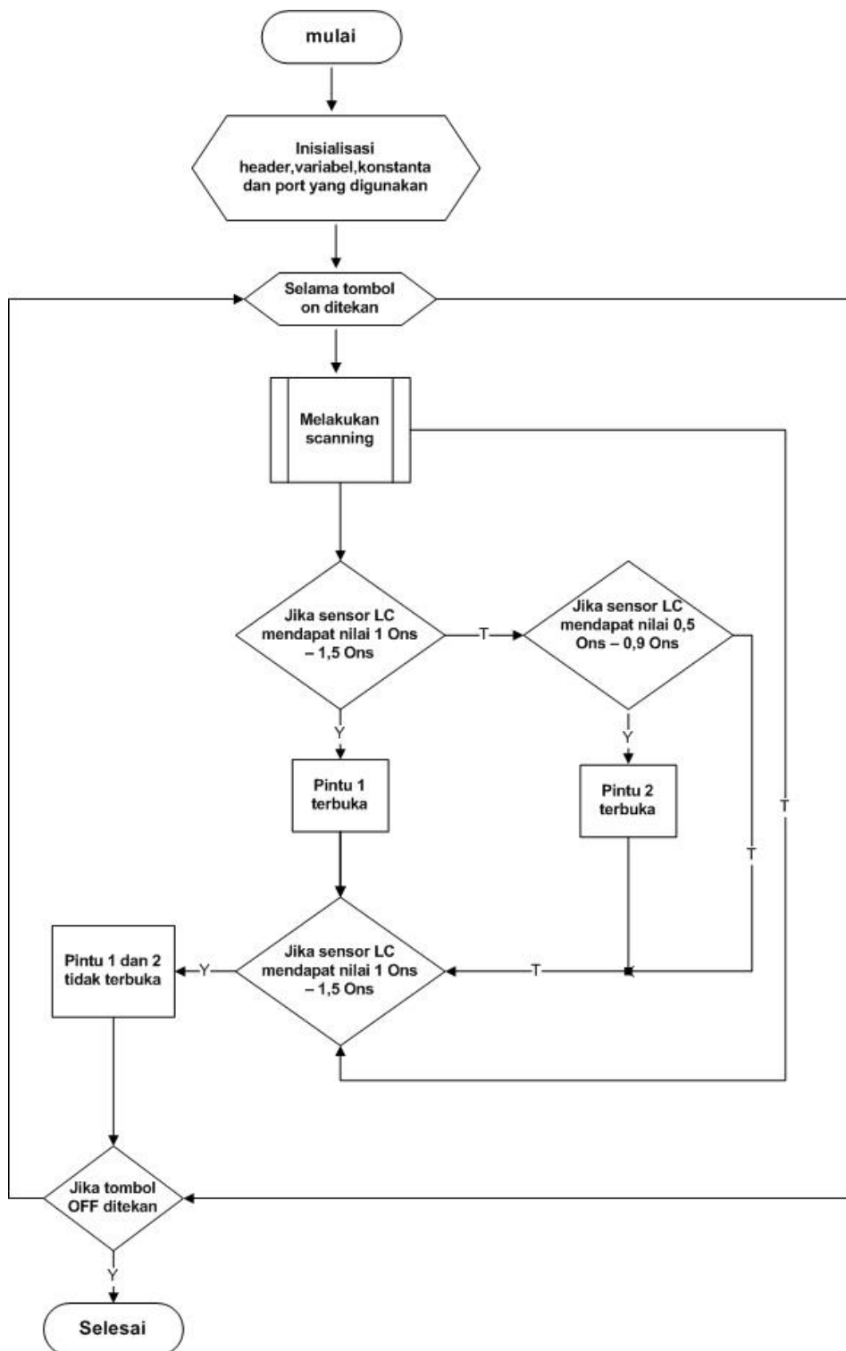
Gambar IV. 5 Flowchart Rancang Bangun Timbangan Otomatis Pensortir Udang Windu.
