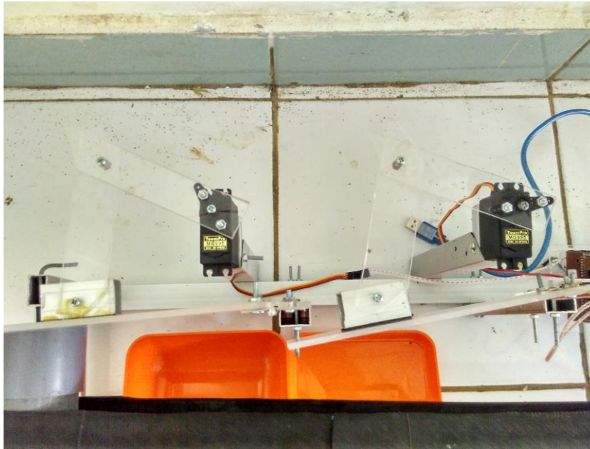
Gambar V. 16 Pintu 1 dan 2 Dalam Keadaan Tertutup.
