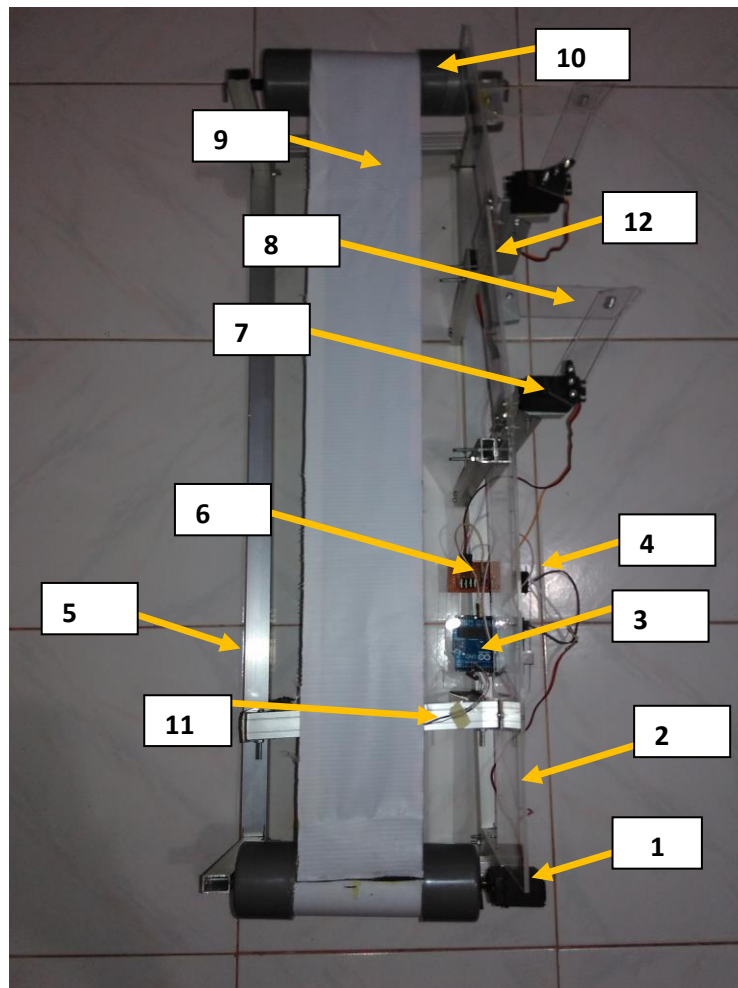
Gambar IV. 2 Rancangan Bentuk Fisik Timbangan.
