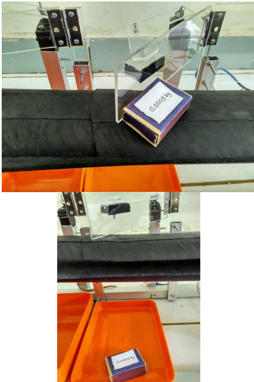
Gambar V. 7 Pensortiran pada Berat 0,0009 Kg (0,9 gram).
