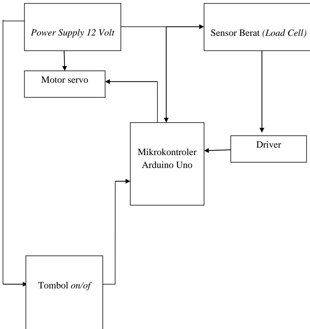
Gambar IV. 1 Diagram Blok Rancang Bangun Timbangan Otomatis Pensortir Udang Windu.
