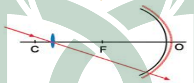
Gambar 2.6: Sinar-sinar istimewa pada lensa cekung
