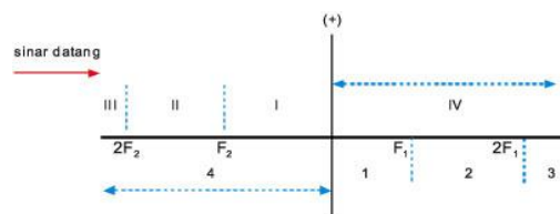
Gambar 2.17: Penomoran ruang pada lensa tipis
