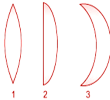
Gambar 2.14 Macam-macam lensa cekung (4) bikonkaf, (2) plankonkaf, (3) konveks Konkaf.
