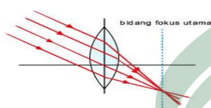
Gambar 2.11: Lensa cembung bersifat Konvergen (mengumpulkan cahaya)
