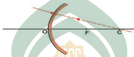
Gambar 2.7: Sinar-sinar istimewa pada lensa cembung
