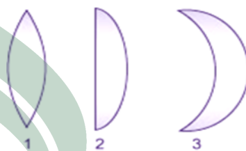
Gambar 2.12: Macam-macam lensa cembung (1) bikonveks (2) plankonveks (3) konkaf konveks
