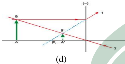
Gambar 2.18: (a), (b), (c), dan (d) Pelukisan bayangan pada lensa tipis
