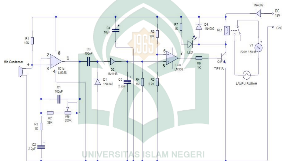
Gambar IV.4. Rangkaian Sensor Suara (Dyan Laksma, 2013)
