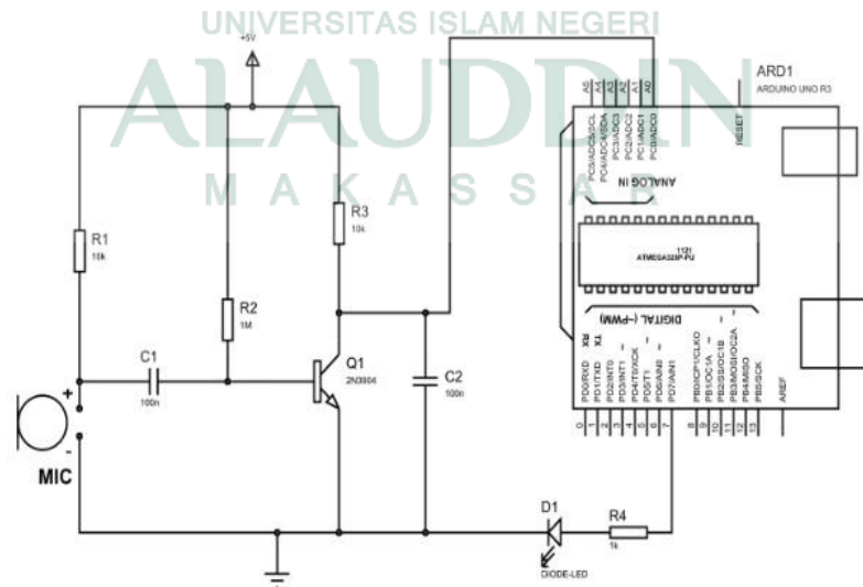
Gambar IV.6. Skematik Sistem
