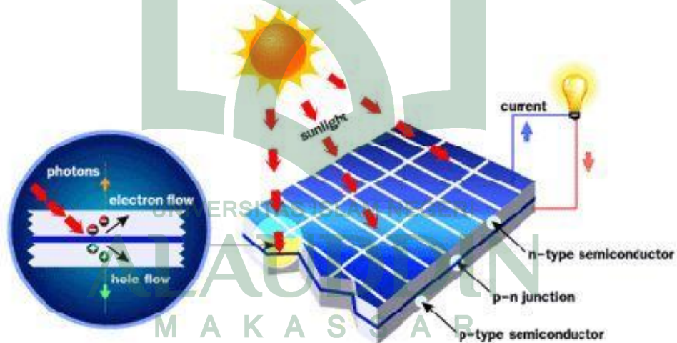
Gambar II 2. Ilustrasi cara kerja sel surya dengan prinsip p-n junction.
