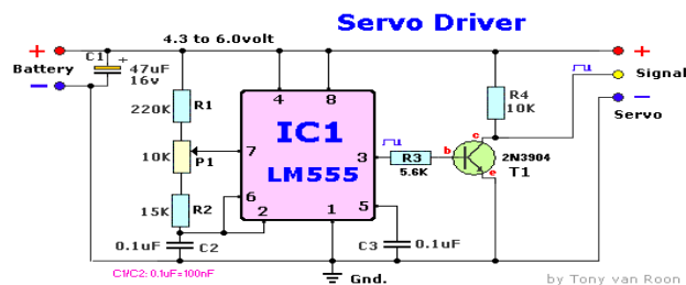
Gambar IV 7. Rangkaian Motor Servo (Yudi, 2015 ).
