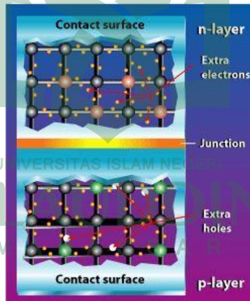
Gambar II 1. Junction antara semikonduktor tipe-p (kelebihan hole) dan tipe-n (kelebihan elektron). (Gambar : eere.energy.gov)
