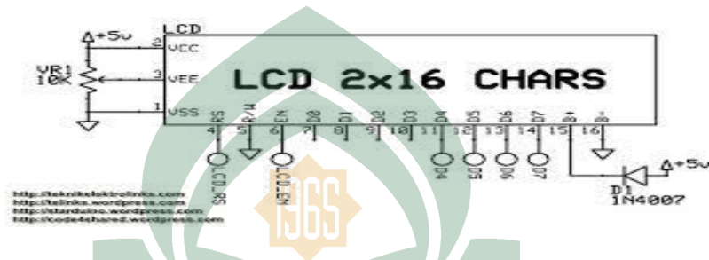
Gambar IV 8. Rangkaian Lcd (Chandra, 2015).
