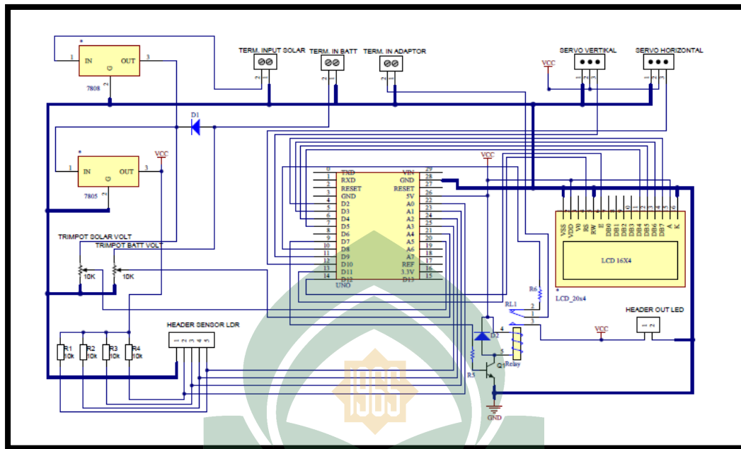
Gambar IV 4. Skema sistem
