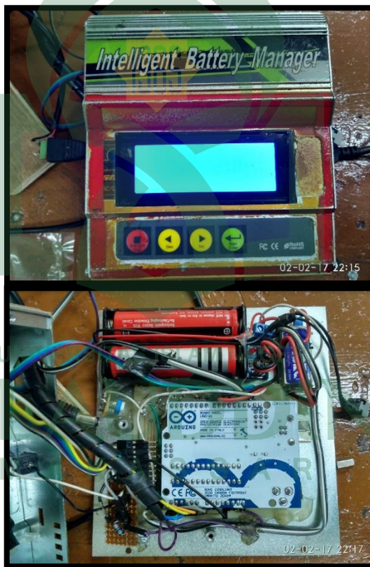
Gambar V 2. Bentuk fisik dari rangkaian Arduino UNO pada kotak kontrol .
