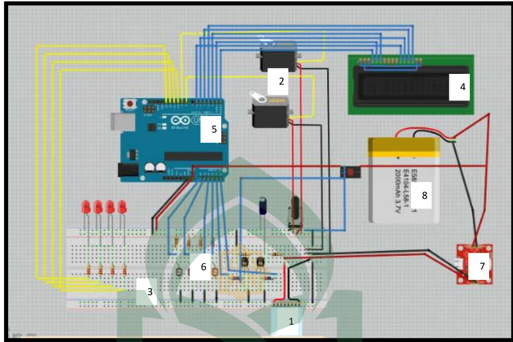
Gambar IV 5 Gambar rangkaian Fisik
