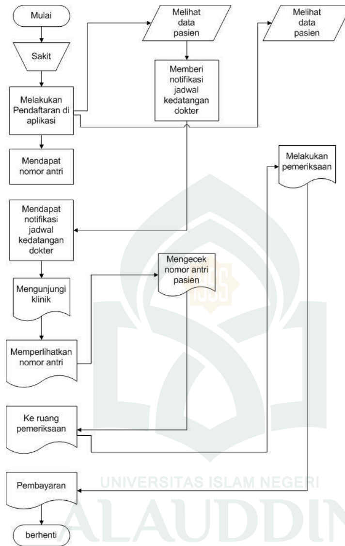
Gambar IV- 2. Flow Map Diagram pada Sistem yang diusulkan
