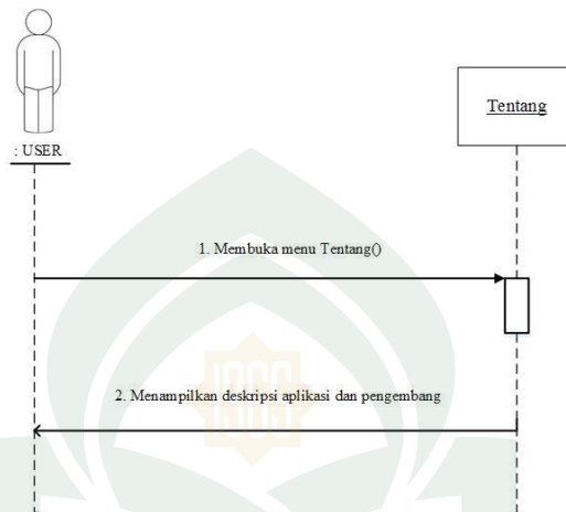
Gambar IV- 10. Sequence Diagram Membuka Menu Tentang
