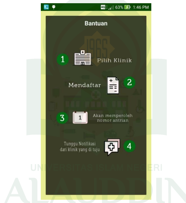
Gambar V- 6. Antarmuka Bantuan
