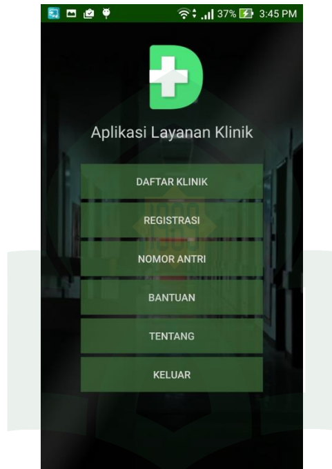
Gambar V- 2. Antarmuka Home
