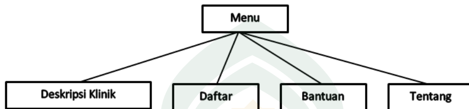
Gambar IV- 13. Struktur Navigasi
