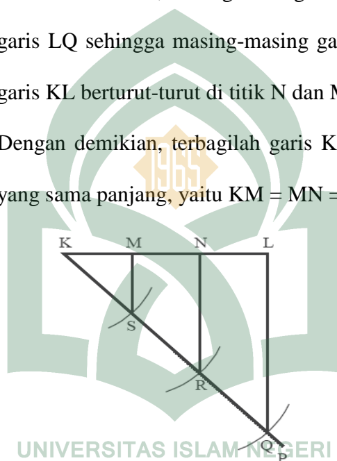
Gambar 11: cara membagi sebuah garis
