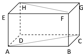
Gambar 5: dua garis bersilangan
