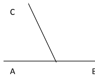
Gambar 17: sudut yang saling bersuplemen
