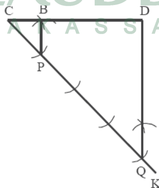
Gambar 13 : cara membagi garis menjadi dua bagian dengan perbandingan 1 : 3
