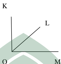
Gamabar 18: sudut yang saling berpenyiku
