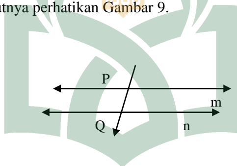
Gambar 9: dua garis sejajar yang dipotong oleh sebuah garis lurus
