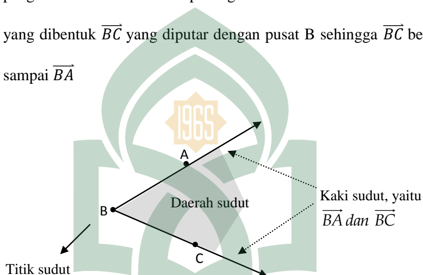
Gambar 15: sudut
