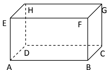
Gambar 3: dua garis saling berpotongan
