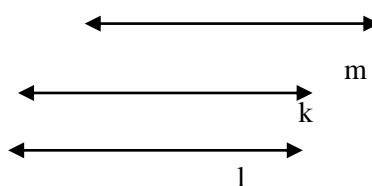
Gambar 10: 3 buah garis lurus yang saling sejajar
