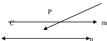
Gambar 8: satu titik di luar sebuah garis yang ditarik pada satu garis sejajar
