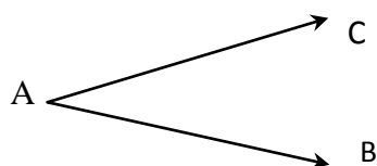
Gambar 19: Sudut BAC
