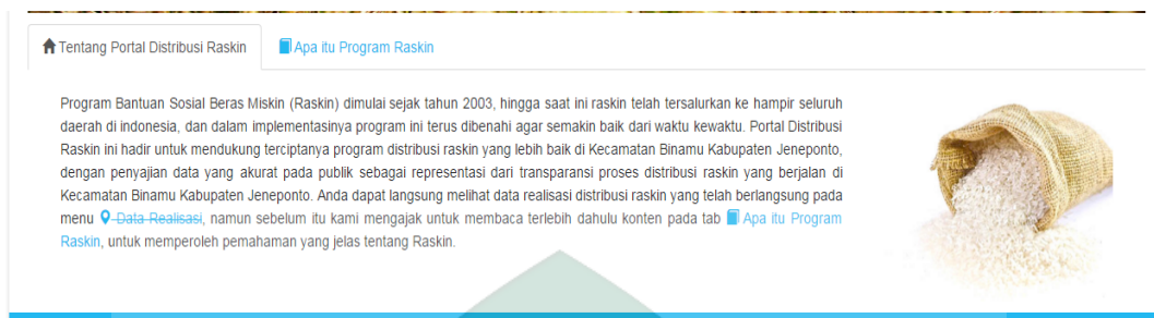
Gambar V.2.Antarmuka Sub Menu 1
