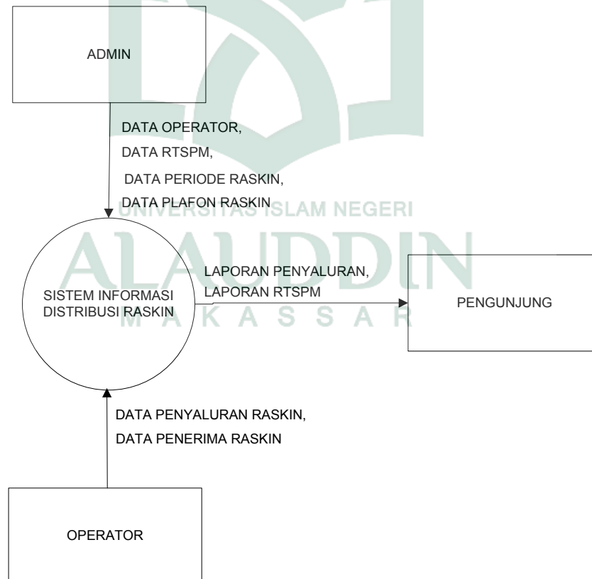
Gambar IV.3. Konteks Diagram
