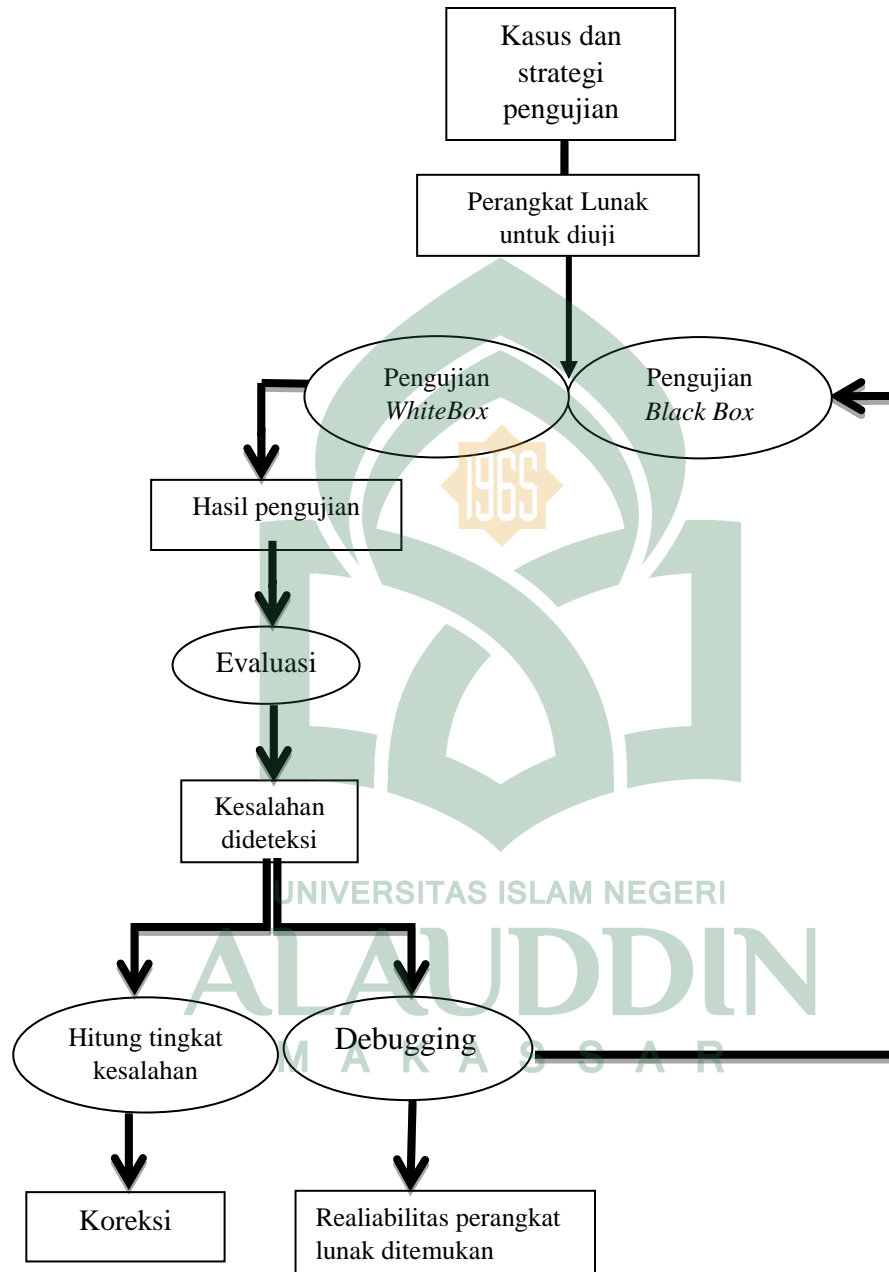
Gambar III.1 Skenario pengujian perangkat lunak terstruktur
