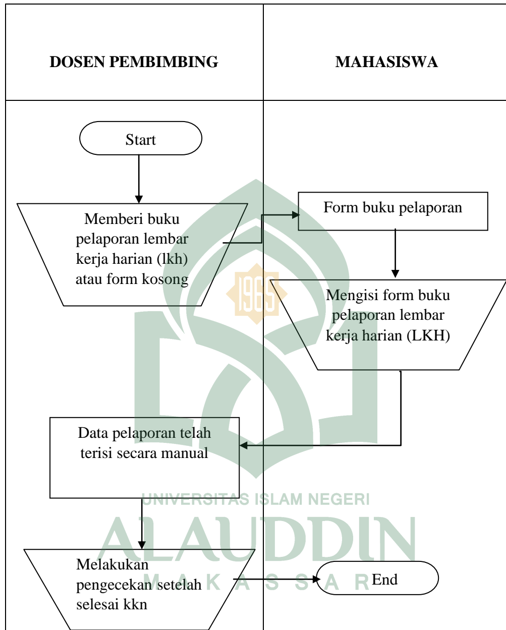
Gambar IV.1 Flowmap Sistem yang sedang berjalan
