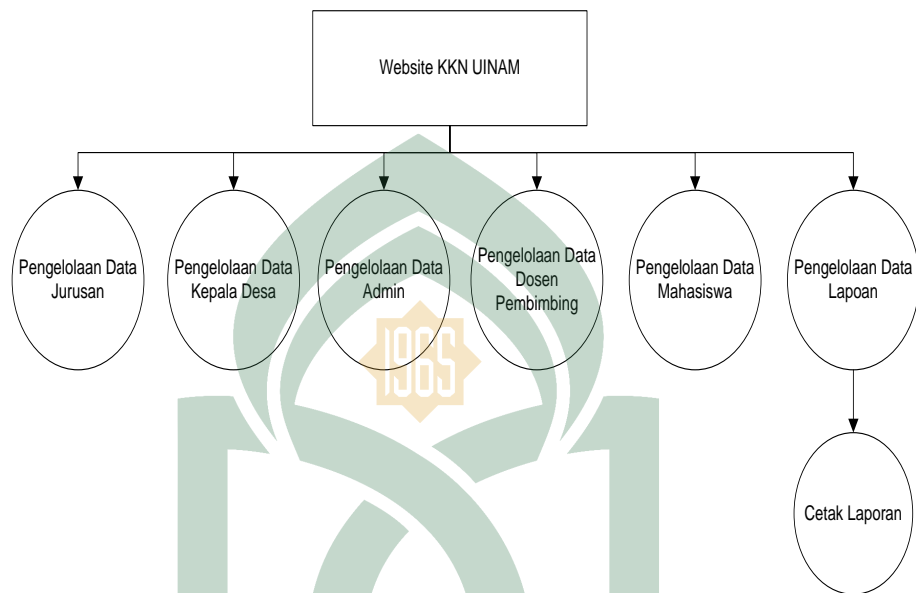
Gambar IV.9. Diagram Berjenjang
