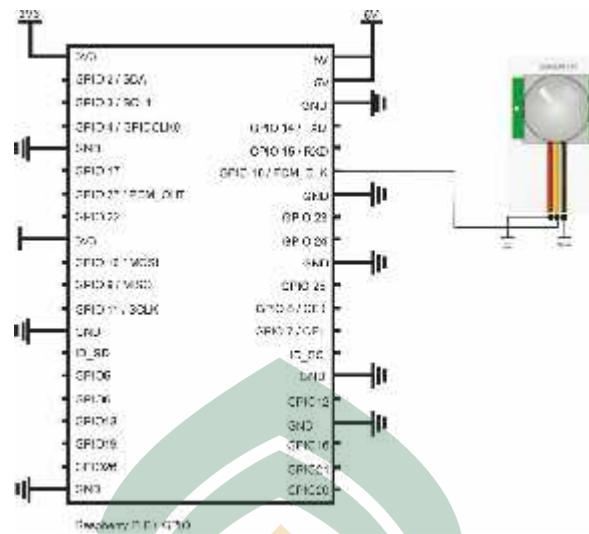
Gambar. IV.2 Skema rangkaian sensor PIR
