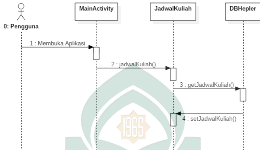
Gambar IV. 8. Sequence Diagram untuk Membuka Jadwal Kelas
