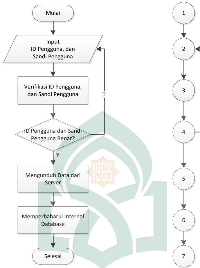
Gambar V. 16. Pengujian Fungsi Login
