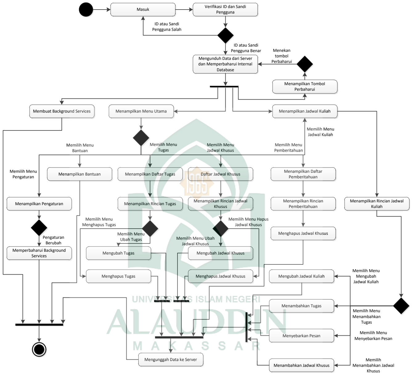
Gambar IV. 12. Activity Diagram Class Reminder untuk Dosen
