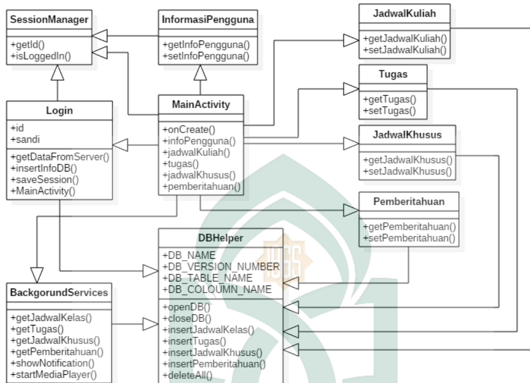
Gambar IV. 5. Class Diagram Sistem yang Diusulkan
