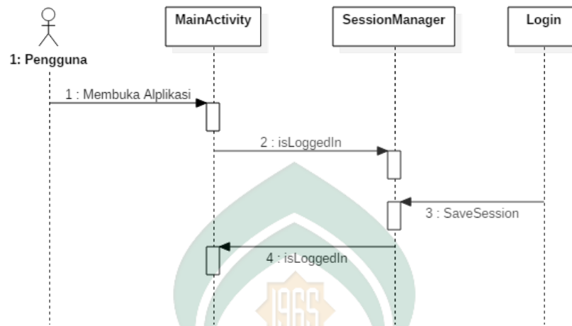
Gambar IV. 6. Sequence Diagram untuk Melakukan Login
