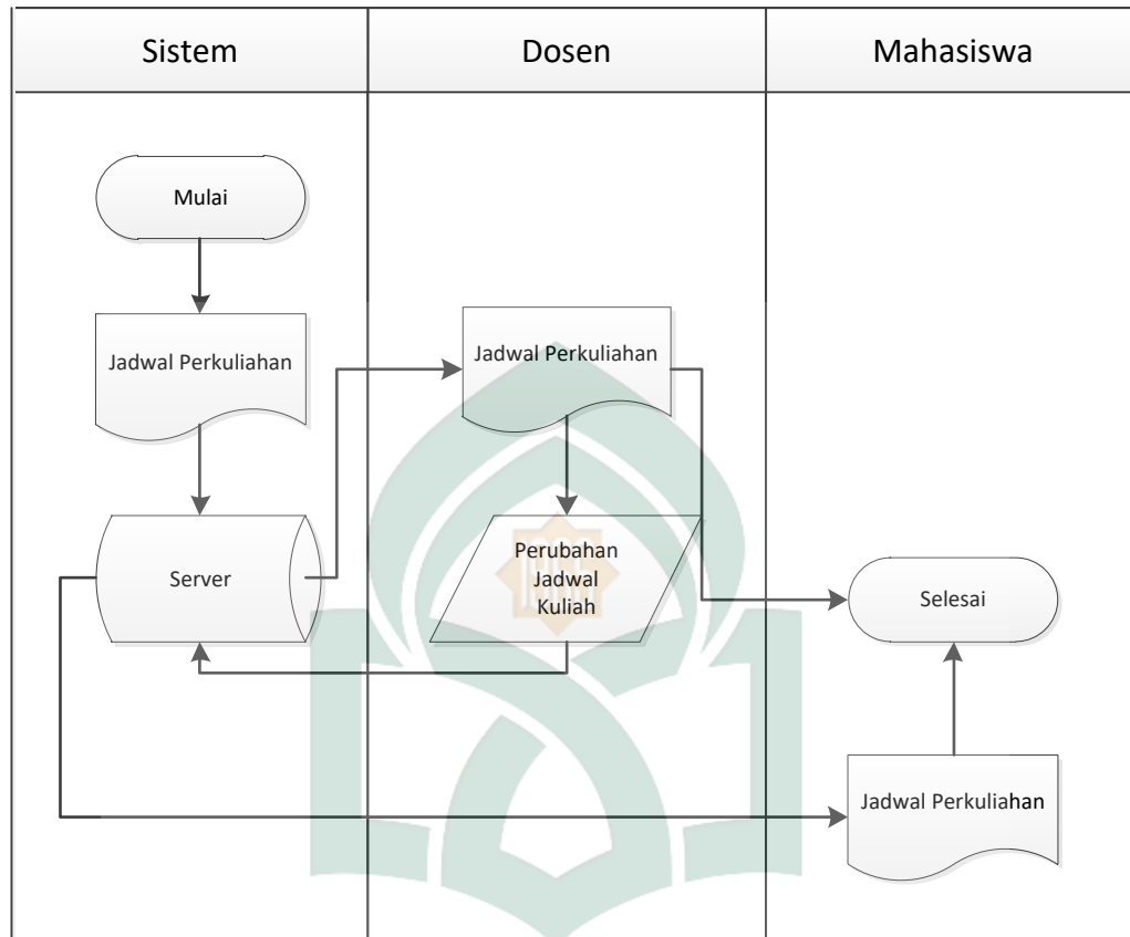
Gambar IV. 2. Flowmap Diagram untuk Sistem yang Diusulkan
