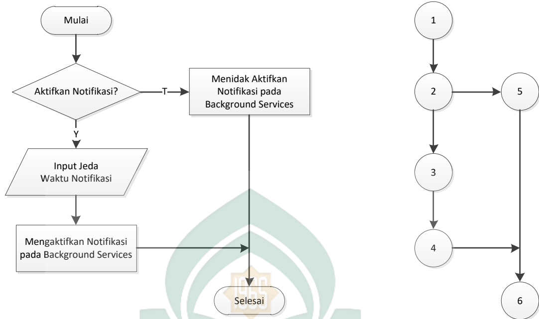
Gambar V. 21. Pengujian Fungsi Pengaturan
