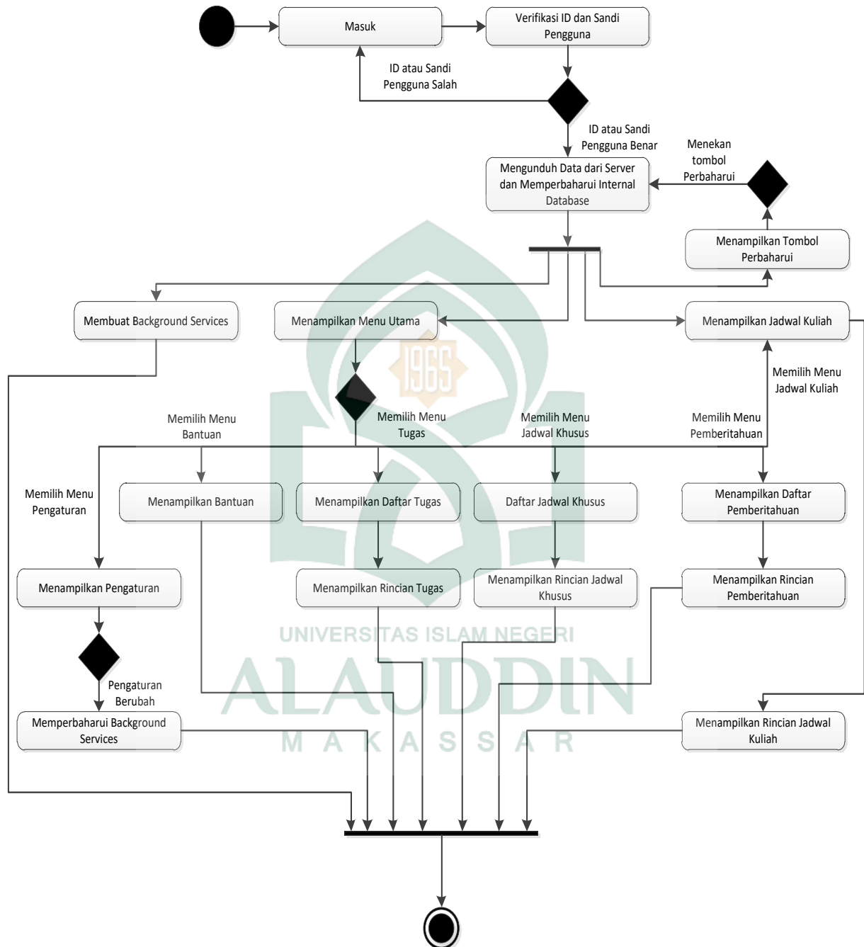
Gambar IV. 13. Activity Diagram Class Reminder untuk Mahasiswa
