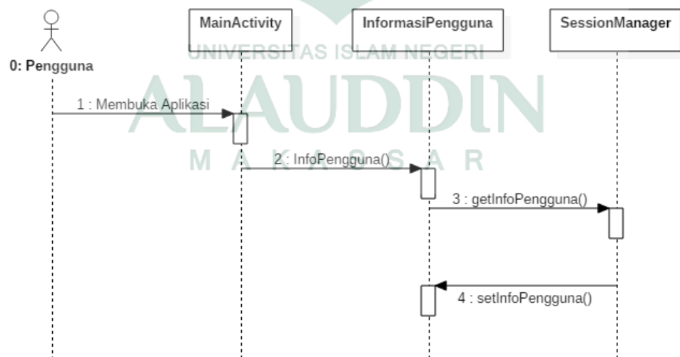
Gambar IV. 7. : Sequence Diagram untuk Membuka Informasi Pengguna
