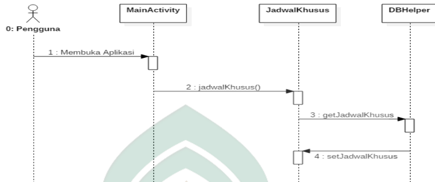
Gambar IV. 10. Sequence Diagram untuk Membuka Jadwal Khusus
