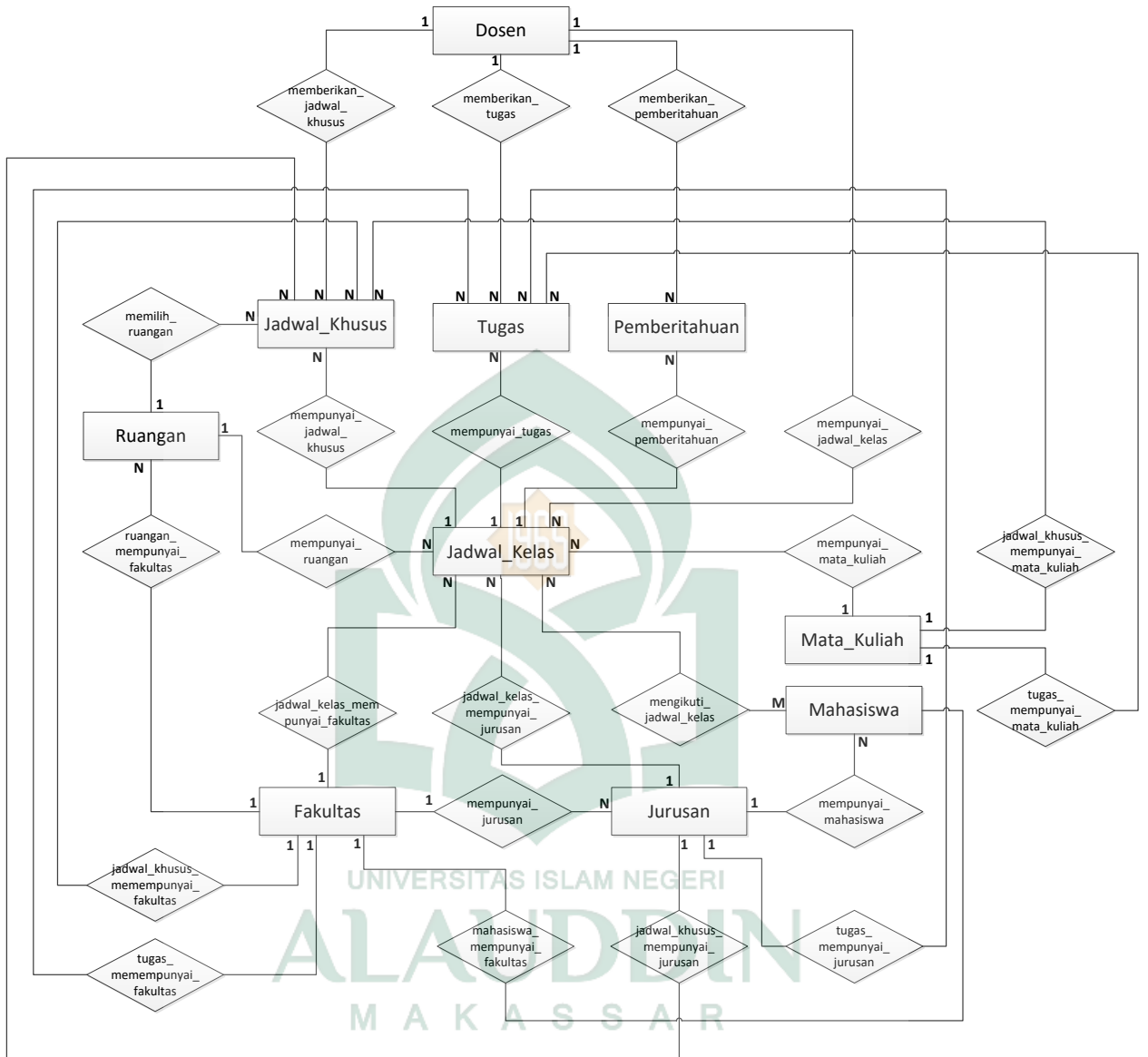
Gambar IV. 3. ERD pada server
