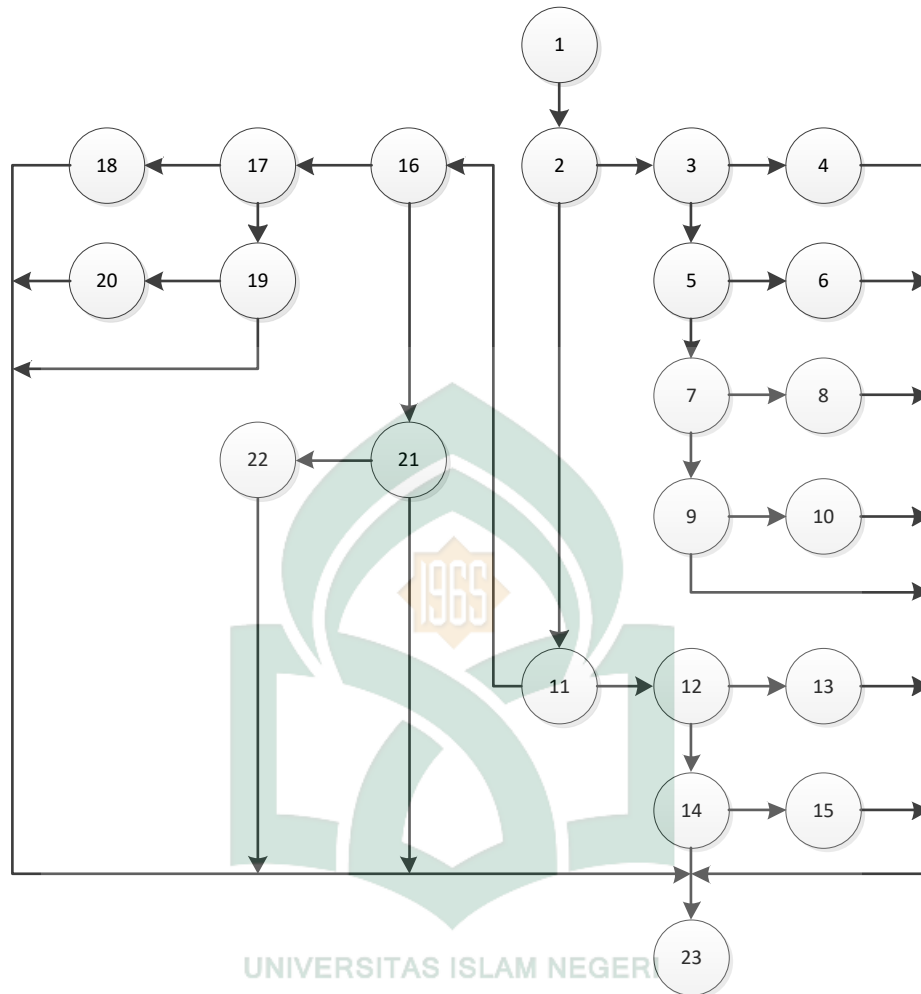
Gambar V. 19. Pengujian Fungsi Tambah, Ubah dan Hapus.
