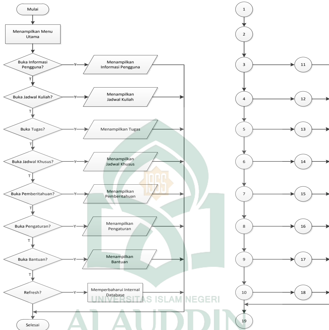
Gambar V. 17. Pengujian Aplikasi Umum
