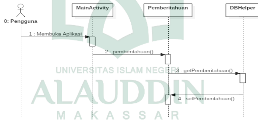
Gambar IV. 11. Sequence Diagram untuk Membuka Pemberitahuan
