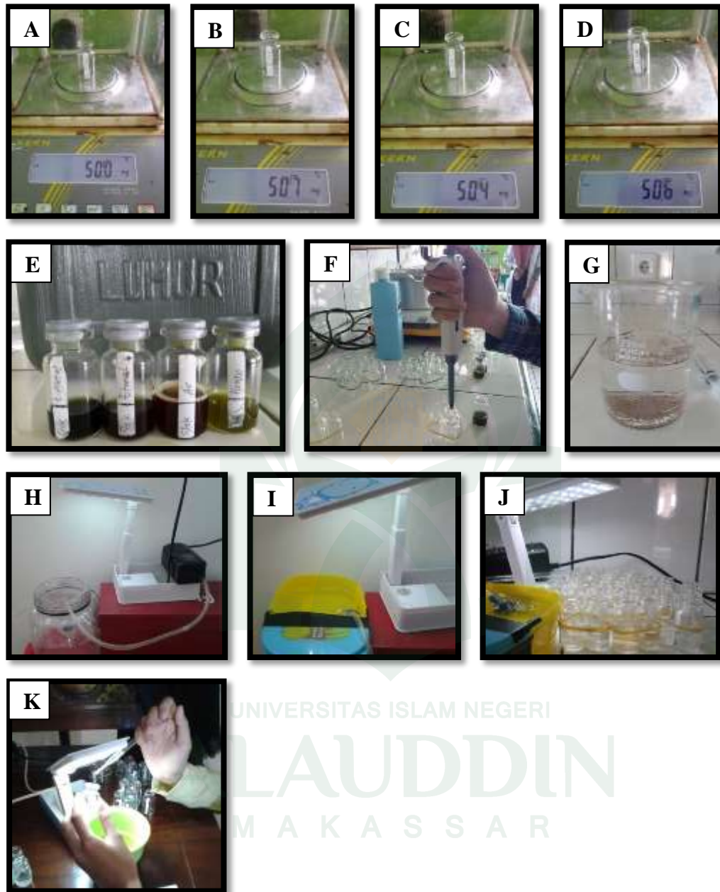
Gambar 4. Pengujian BSLT pada ekstrak
