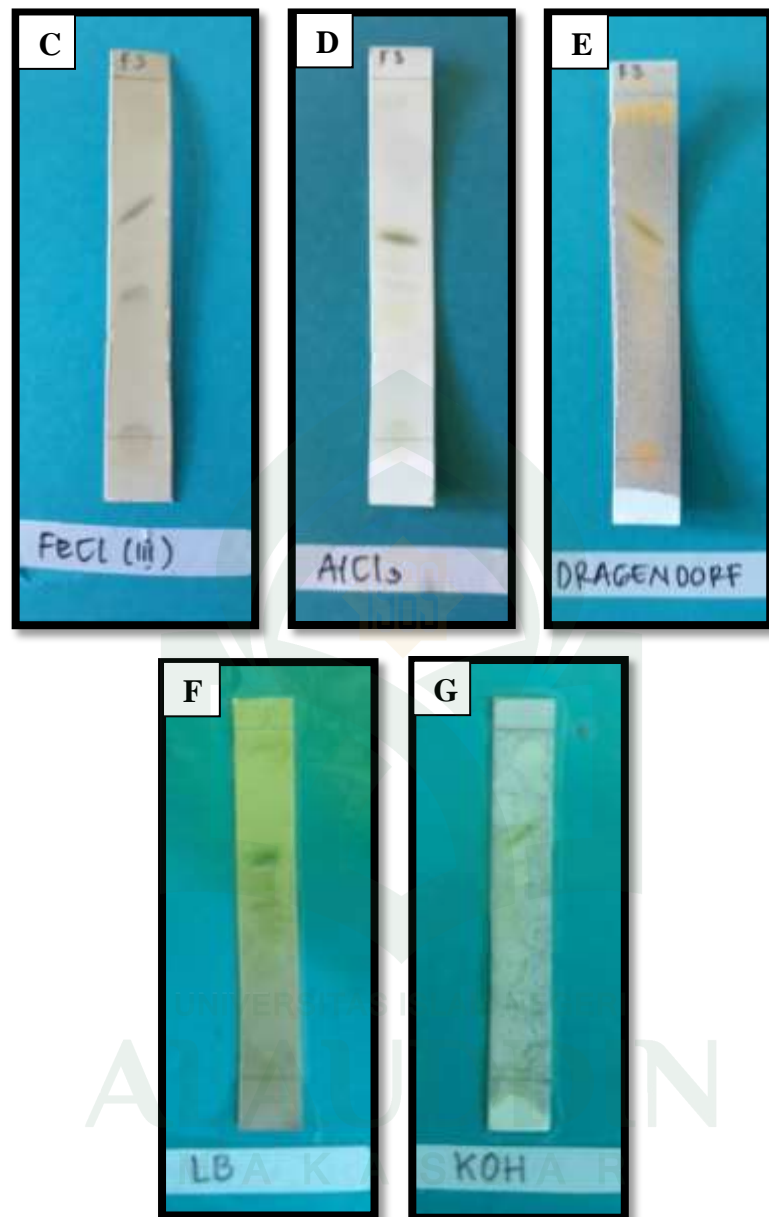
Gambar 9. Identifikasi golongan senyawa
