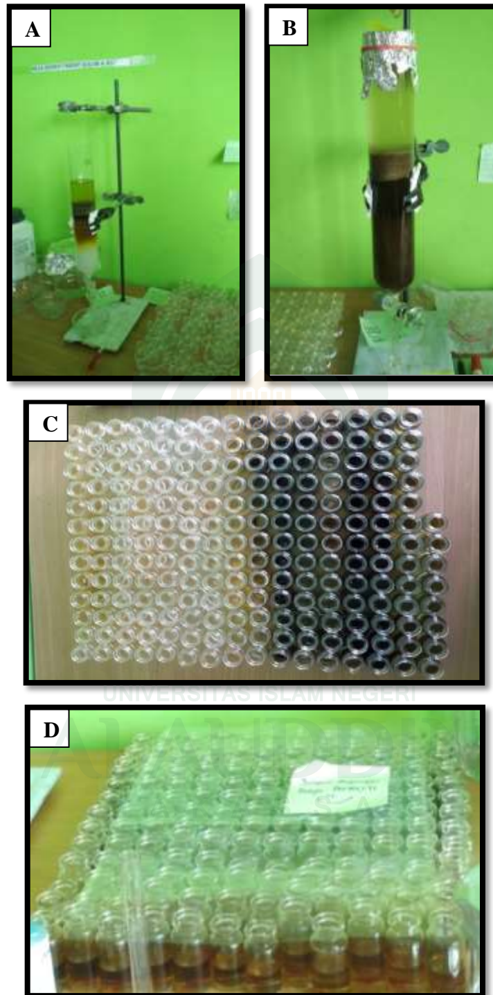
Gambar 6. Proses koromatografi kolom
