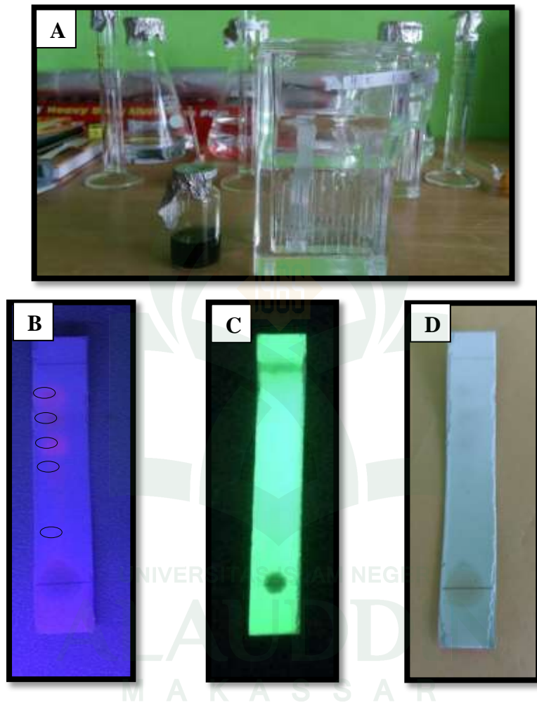
Gambar 5. Kromatografi lapis tipis
