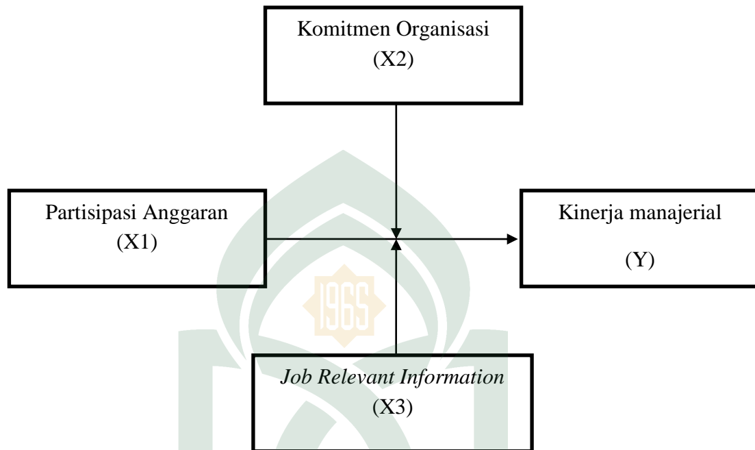
Gambar 2.1 Rerangka Pikir
