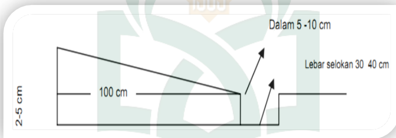
Gambar 49. Kemiringan lantai kandang
