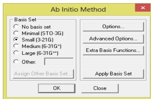
Gambar III.2. Panel Optimasi Ab Initio menggunakan program Hyperchem
