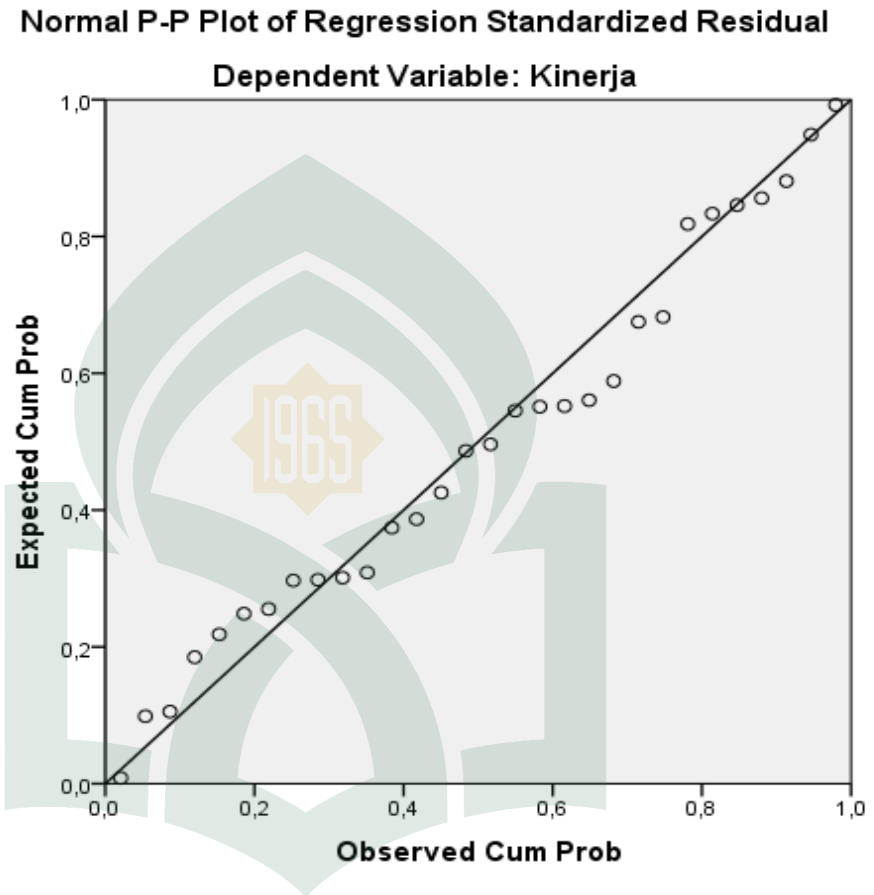
Gambar 4.4 P-Plot Hasil Uji Normalitas
