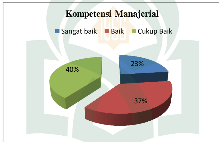
Gambar 4.2 Deskripsi Presentase Kompetensi Manajerial
