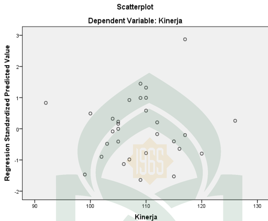
Gambar 4.5 Uji Heteroskedastisitas
