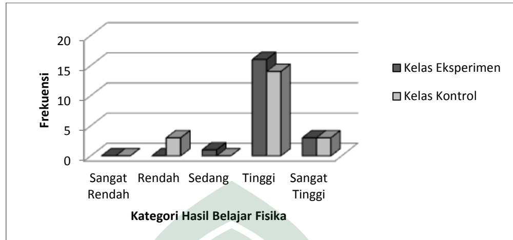
Gambar 4.1: Histogram Kategori Nilai Hasil Belajar Fisika
