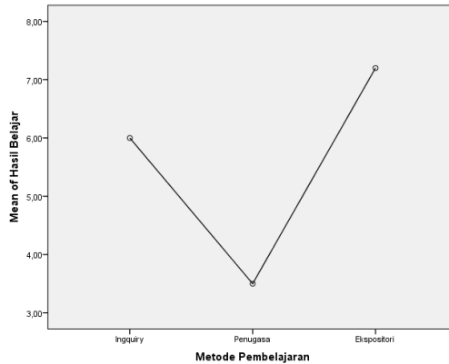
Gambar 7.1. Rata-Rata Kemampuan Berpikir Kritis Siswa
