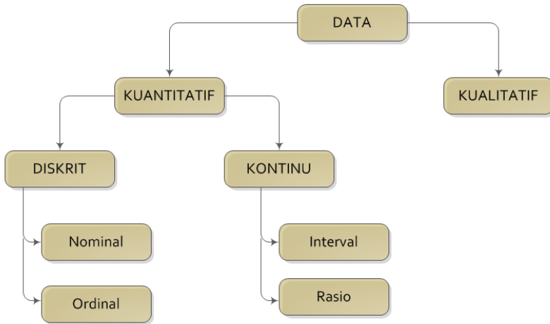
Gambar 2.1. Jenis-Jenis Data
