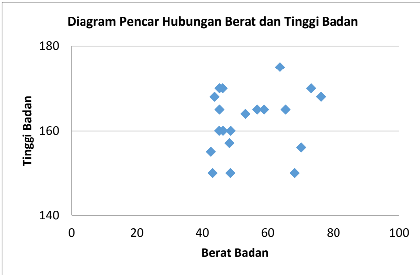
Gambar 2.5. Diagram Pencar Hubungan Antara Berat dan Tinggi Badan Mahasiswa
