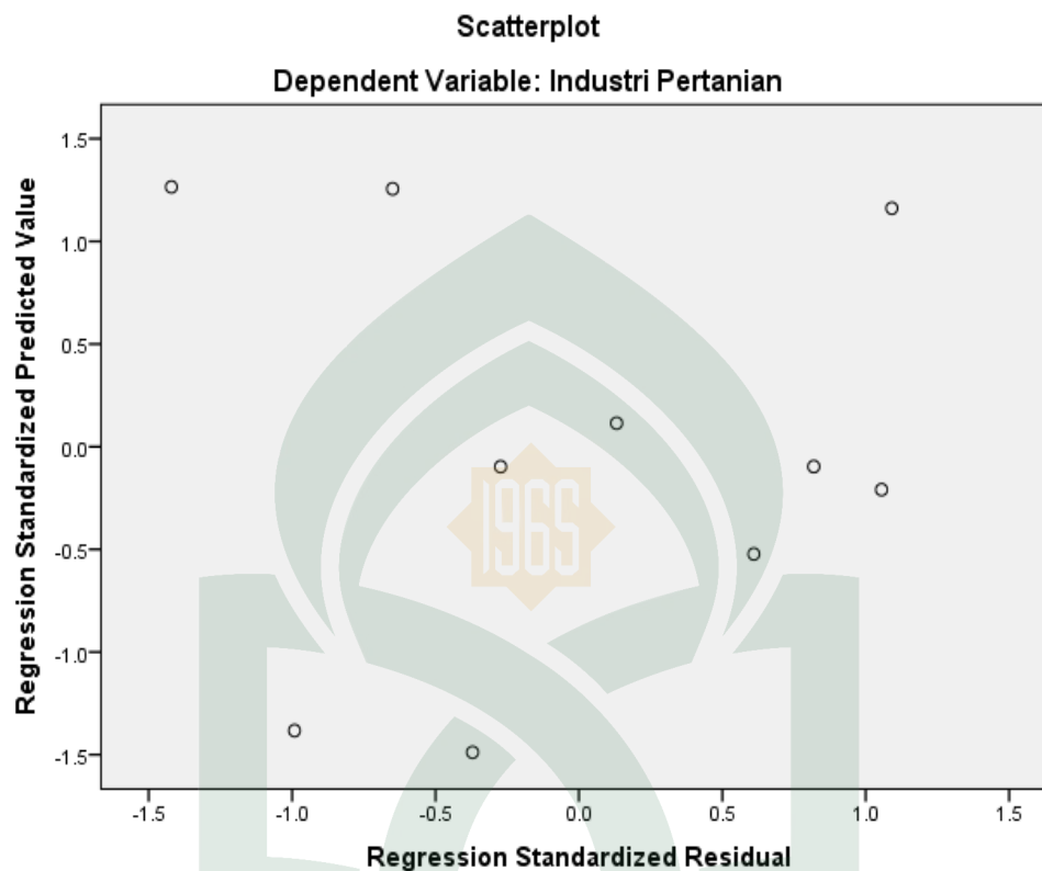
Gambar 4.3 Uji Heteroksedastisitas
