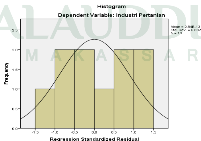
Gambar 4.1 Grafik Histogram
