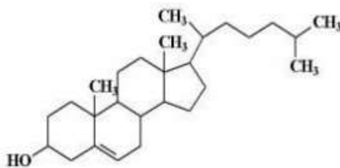
Gambar 2.1 Struktur Kolesterol
