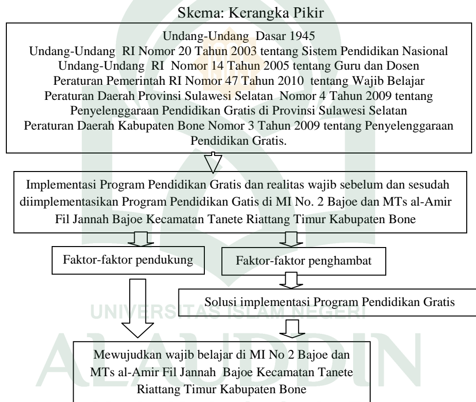
Gambar. 1 . 2 Kerangka Pikir
