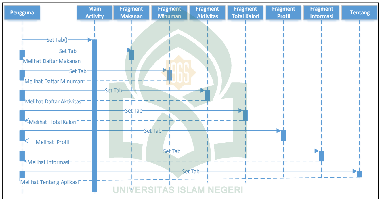
Gambar IV. 5. Sequence Diagram Aplikasi Monitoring Kecukupan Kalori
