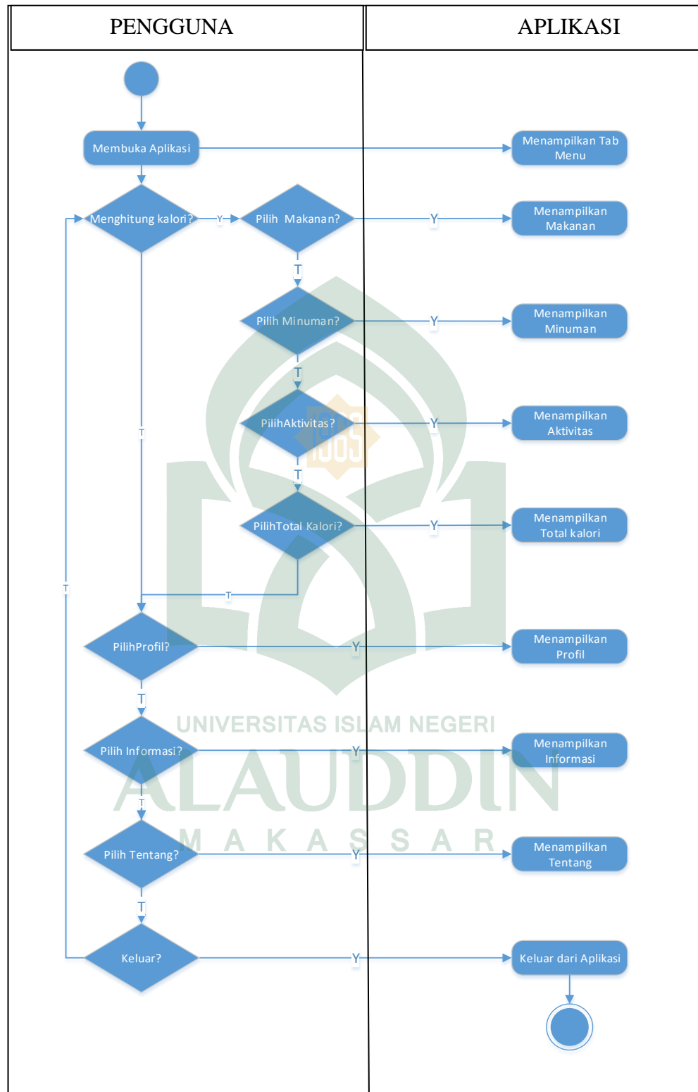
Gambar IV. 6. Activity Diagram Sliding Menu Aplikasi
