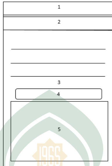
Gambar IV. 12. Desain Antarmuka Menu Total Kalori
