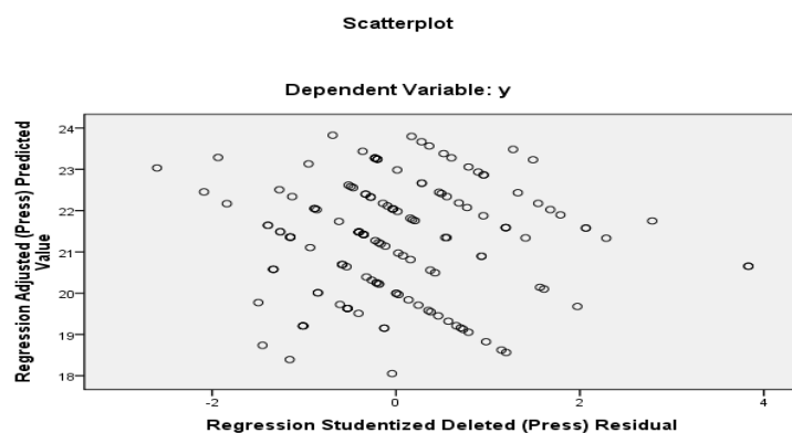
Gambar 4.2 Uji Heteroskedastisitas
