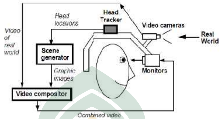
Gambar 2.2 Diagram Opaque HMD. Sumber: Paul M.(2007)
