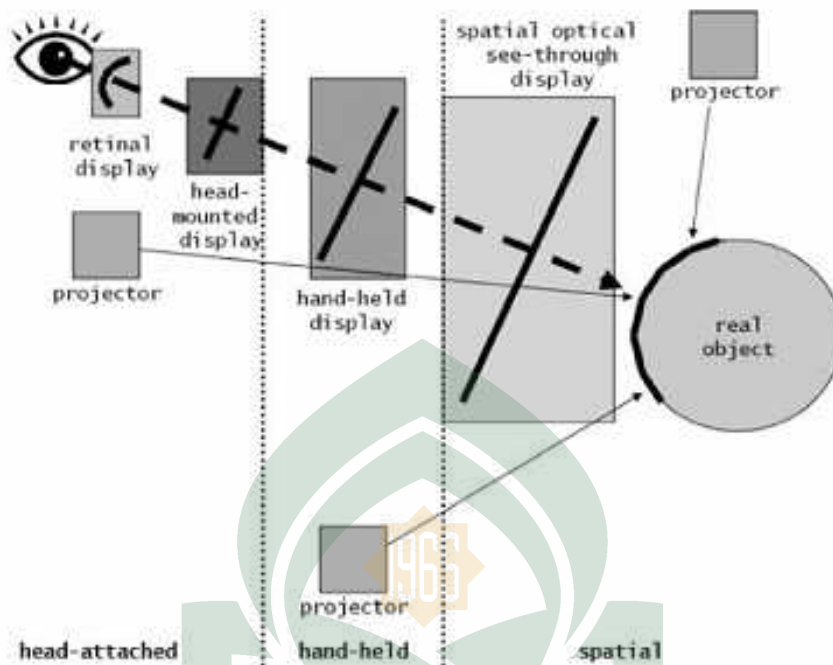
Gambar 2.1 Pembentukan citra untuk display Augmented Reality. Sumber : Paul M.(2007)
