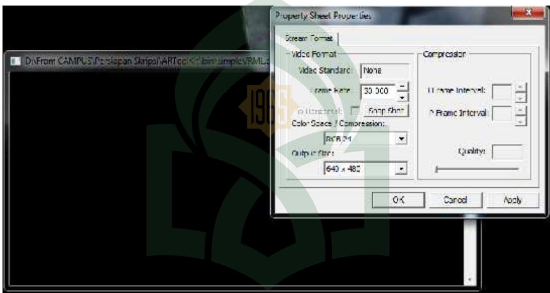
Gambar 5.9 Menjalankan simplevrm.exe
