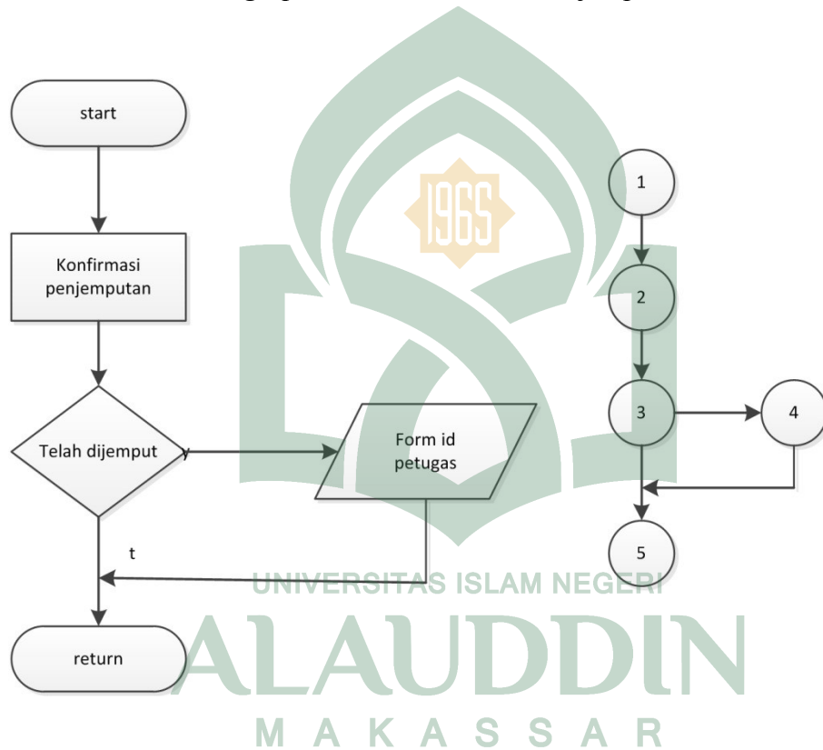
Gambar V.18 Flowchart dan Flowgraph Menu Konfirmasi Penjemputan
