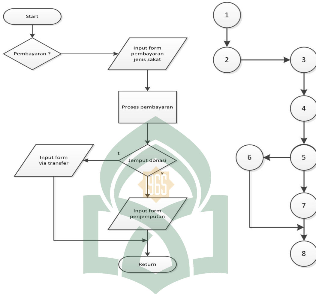
Gambar V.15 Flowchart dan Flowgraph Pembayaran Zakat
