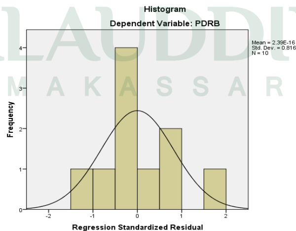
Gambar 4.6: Grafik Histogram
