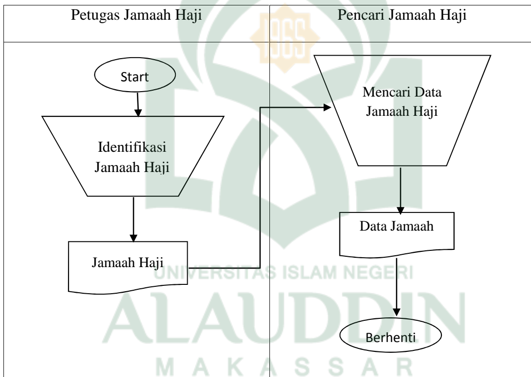
Gambar IV. 1 Sistem yang sedang berjalan
