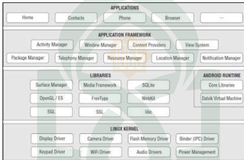
Gambar II.3 Arsitektur Android OS (Nazruddin, 2011)
