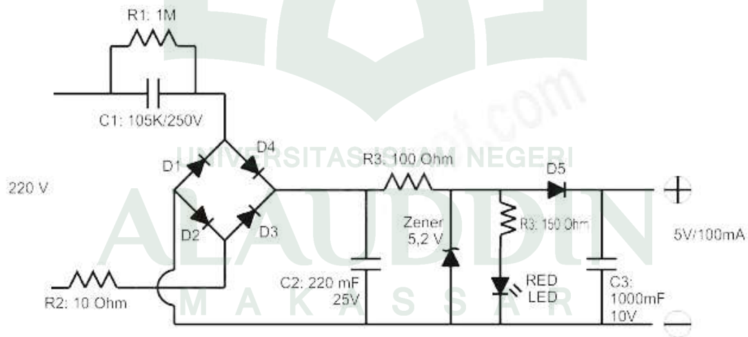
Gambar IV.3 Rangkaian Power Supply (Suhartono, 2015).
