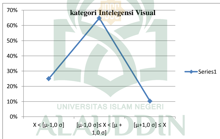
Gambar 4.1 : Diagram Garis Kategori Intelegensi Visual
