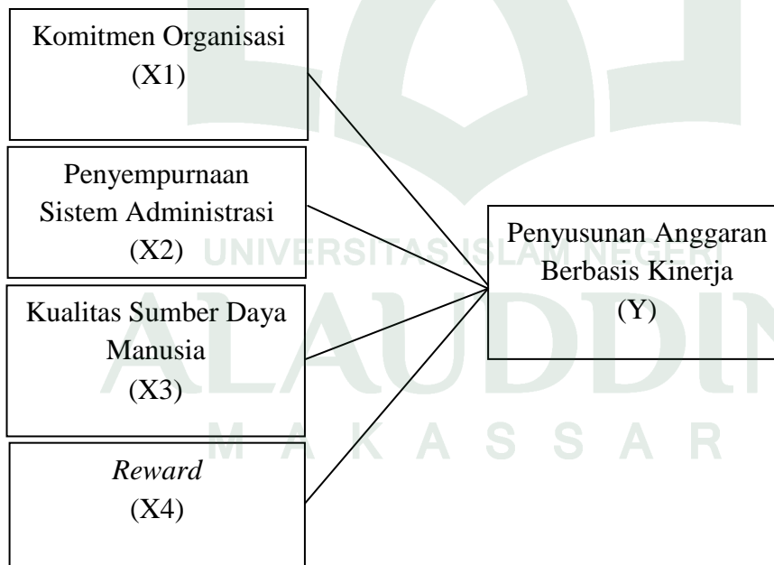
Gambar 2.1 Rerangka Teori
