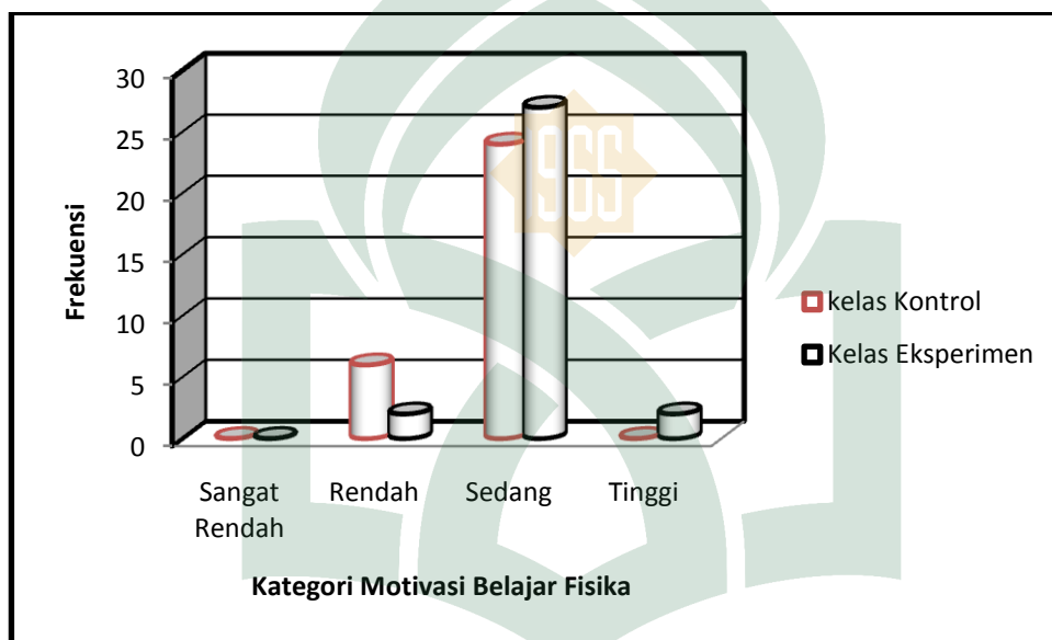
Gambar 4.1: Histogram Kategori Skor Motivasi Belajar Fisika
