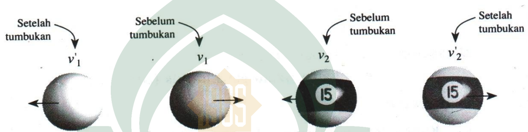
Gambar 1.3 Berlaku Hukum III Newton ketika terjadi tumbukan antara dua buah bola.
