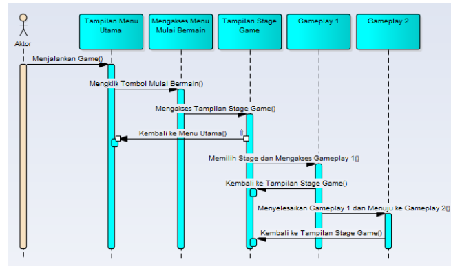
Gambar IV.6 Sequence Diagram Memulai Bermain
