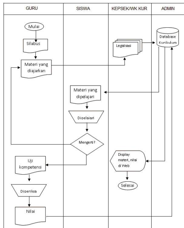
Gambar IV.1 Diagram Flowmap Sistem Yang Sedang Berjalan
