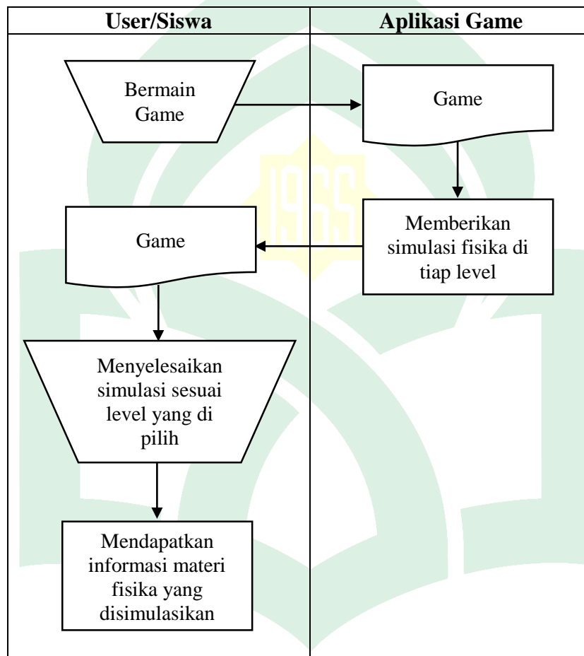
Gambar IV.2 Diagram Flowmap Sistem Yang Diusulkan
