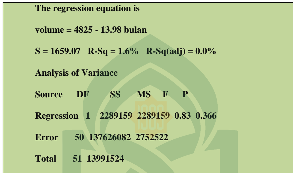
Gambar 4.2 output hasil olahan minitab
