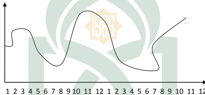
Gambar 2.3. Grafik komponen musiman
