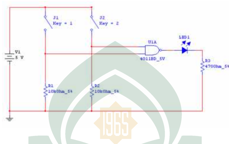
Gambar 2.4. Rangkaian logika NAND menggunakan IC 4011
