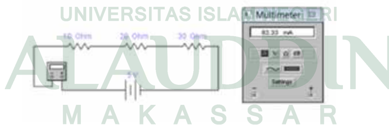
Gambar 2.10 Mengukur Arus
