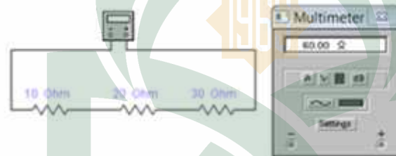
Gambar 2.9 Mengukur R_{\text{Total}} pada Rangkaian Seri
