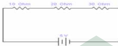
Gambar 2.8 Rangkaian seri
