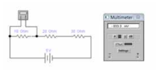
Gambar 2.11 Mengukur Tegangan
