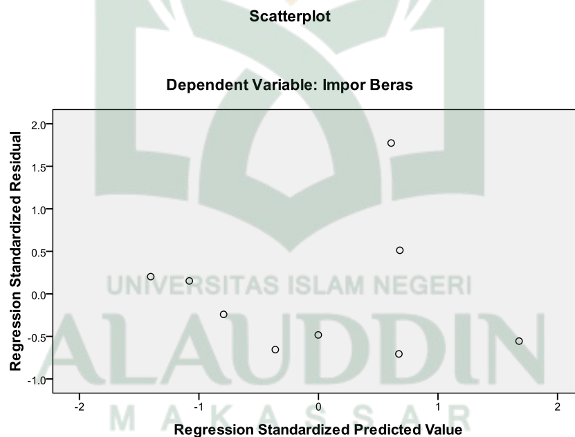
Gambar 4.2 : Grafik Scatterplot
