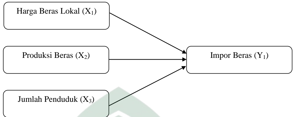
Gambar 1.1 Kerangka Pikir
