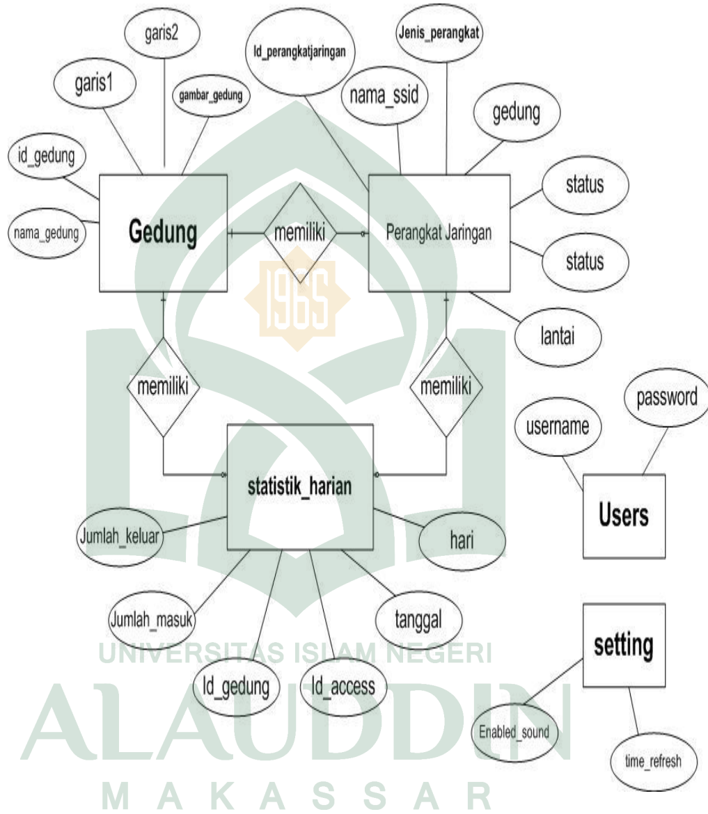
Gambar 4.20 Relasi antar tabel
