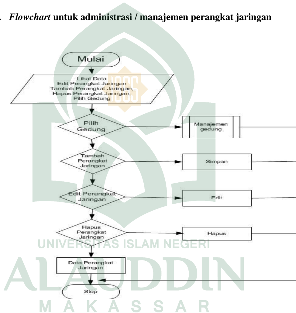
Gambar 4.18 Flowchart Halaman Administrasi Perangkat Jaringan
