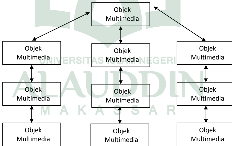
Gambar IV.3 Struktur Menu
