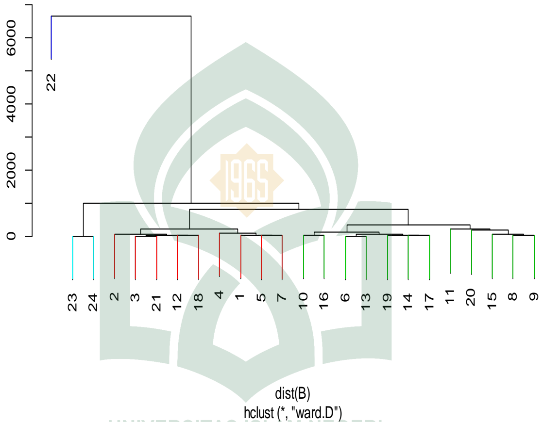
Gambar 4.1. Hasil Dendrogram untuk Metode Ward
