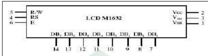
Gambar IV.5 : Pin LCD
