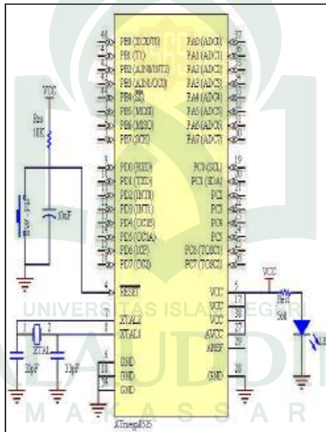
Gambar IV.3 : Rangkaian Sistem Minimum Mikrokontroler Atmega 8538
