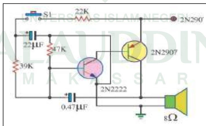
Gambar IV.6 : Rangkaian skematik Sirine
