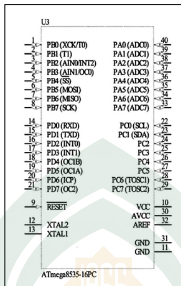
Gambar II.2 : Konfigurasi Pin Mikrokontroler ATmega8535 (Budiharto & Togu Jefri : 2007:54)
