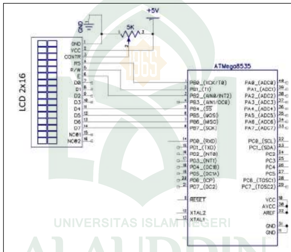
Gambar IV.4 : Rangkaian skematik LCD 2x16
