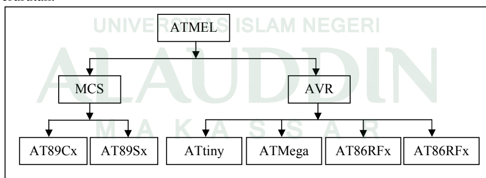
Gambar II.1 : Blok Perkembangan Mikrokontroler ATMEL MCS (Setiawan, 2011)
