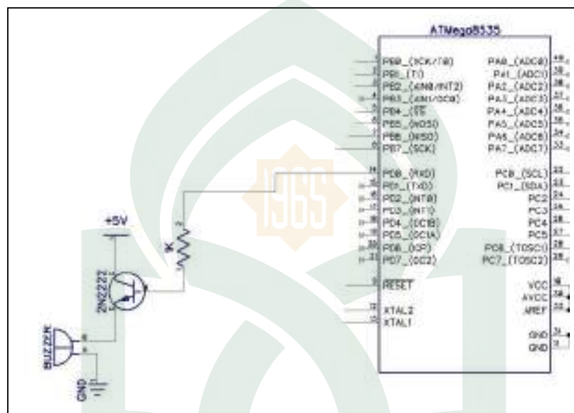
Gambar IV.7 : Rangkaian skematik Sirine pada sistem peringatan
