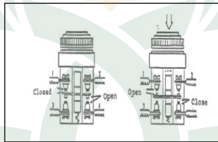
Gambar II.6 : Push button tipe NO dan NC
