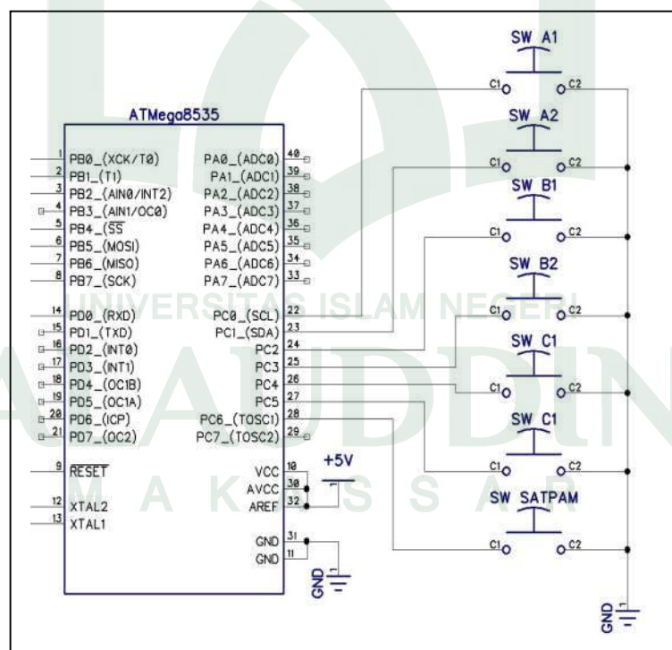
Gambar IV.2 : Rangkain Skematik Push button
