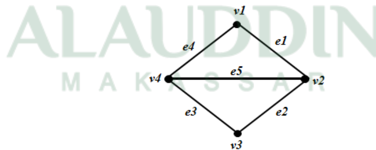
Gambar 2.1 . Sebuah graf
