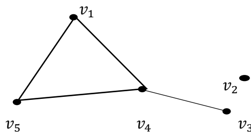
Gambar 2.11. Simpul terpencil
