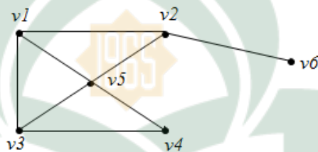
Gambar 2.20. Sebuah graf 29
