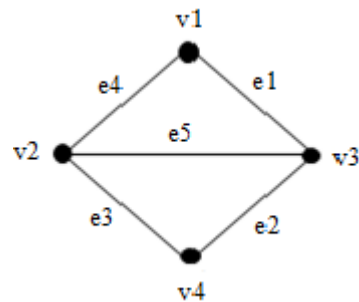
Gambar 2.14. Sebuah graf 24
