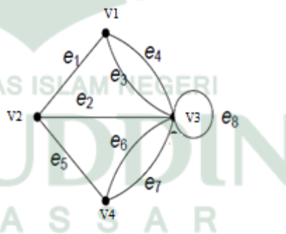
Gambar 2.4. Graf semu
