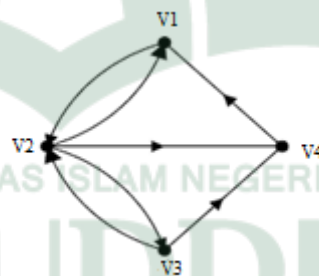
Gambar 2.6. Graf berarah
