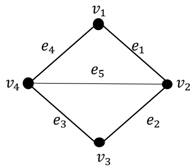
Gambar 2.10. Graf bersisian
