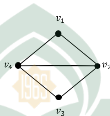
Gambar 2.9. Graf bertetangga 19
