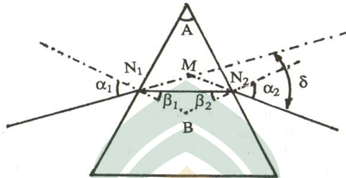
Gambar II.6 : Pembiasan pada prisma
