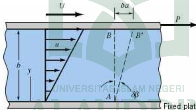
Gambar II.7 : Aliran laminar dari fluida viskos. Pelat di atas dan di bawah fluida masing-masing mempunyai luas A . Viskositas adalah perbandingan dari tegangan geser F/A terhadap laju tegangan v/l . 52
