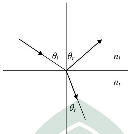
Gambar II.5 Pembiasan pada dua medium yang berbeda. Medium I adalah udara dan medium II adalah kaca.
